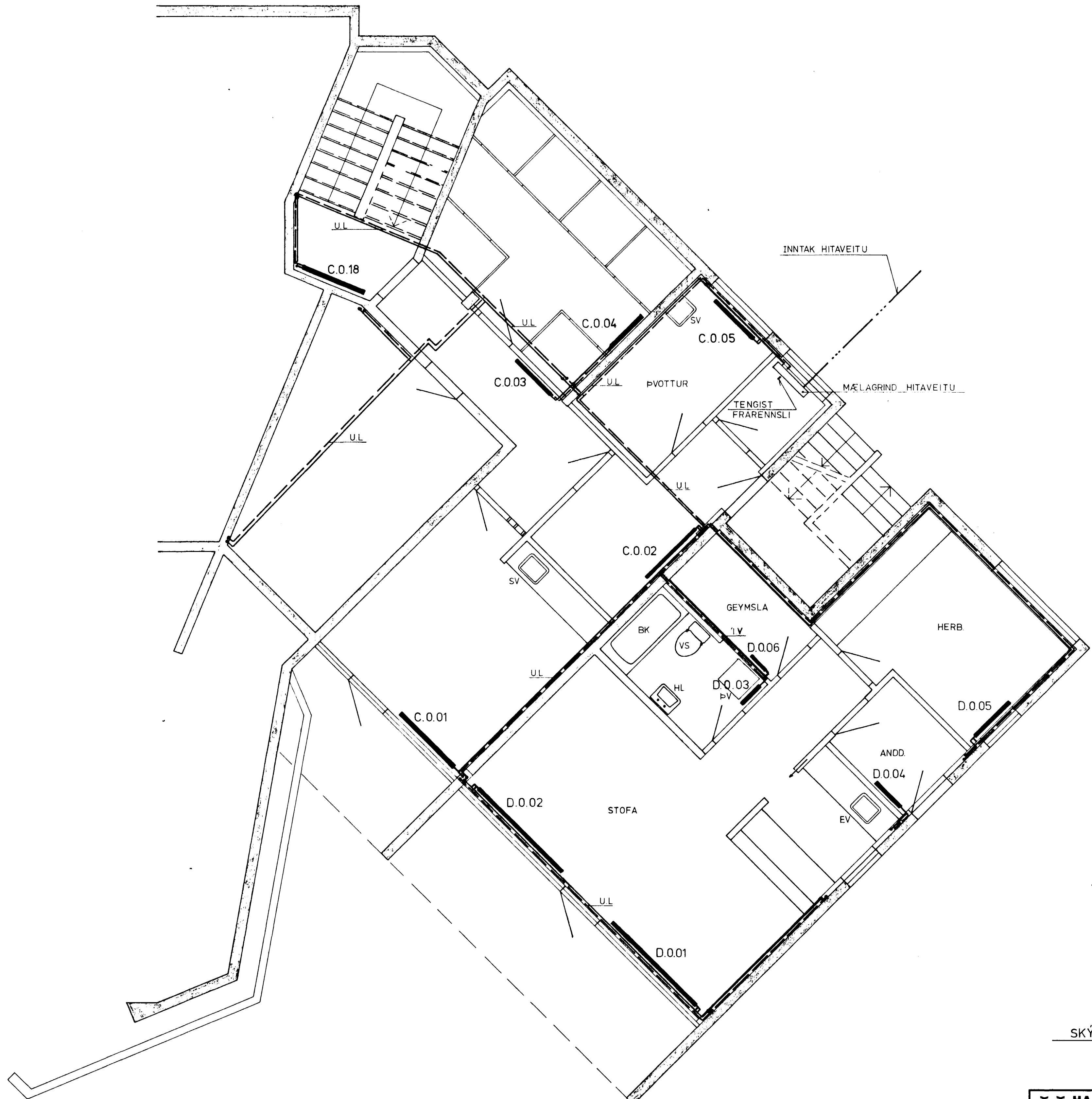
GRUNNMYND KJALLARA 1:50
