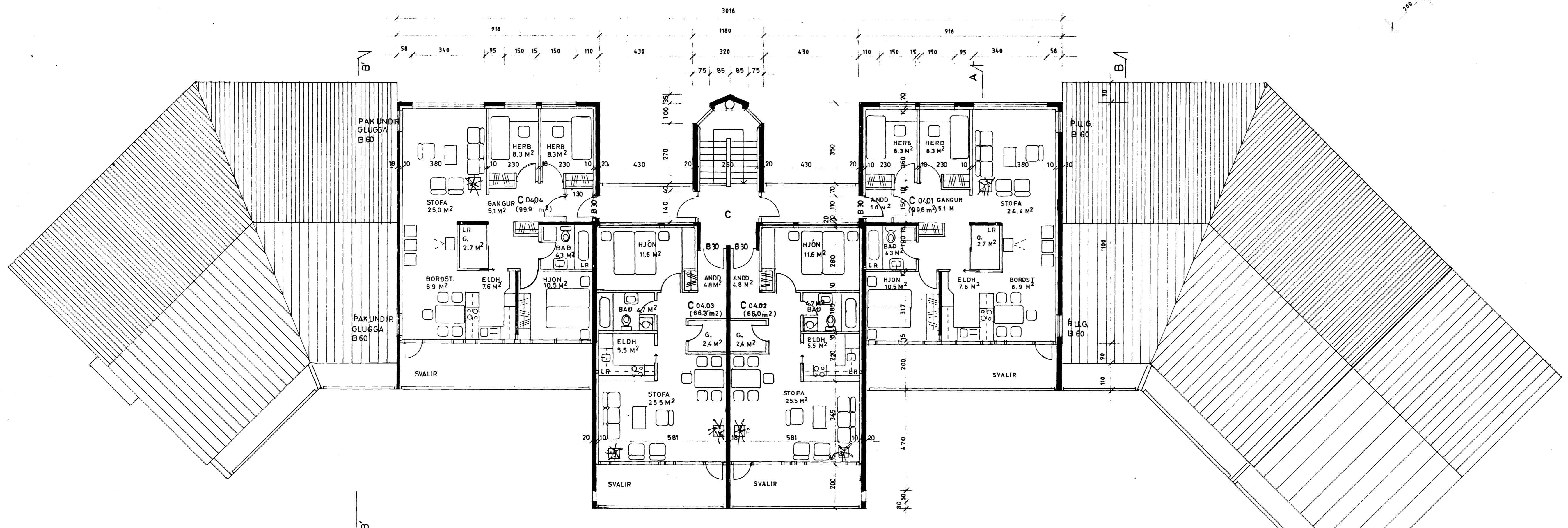
GRUNNMÝND 4. HÆÐAR
