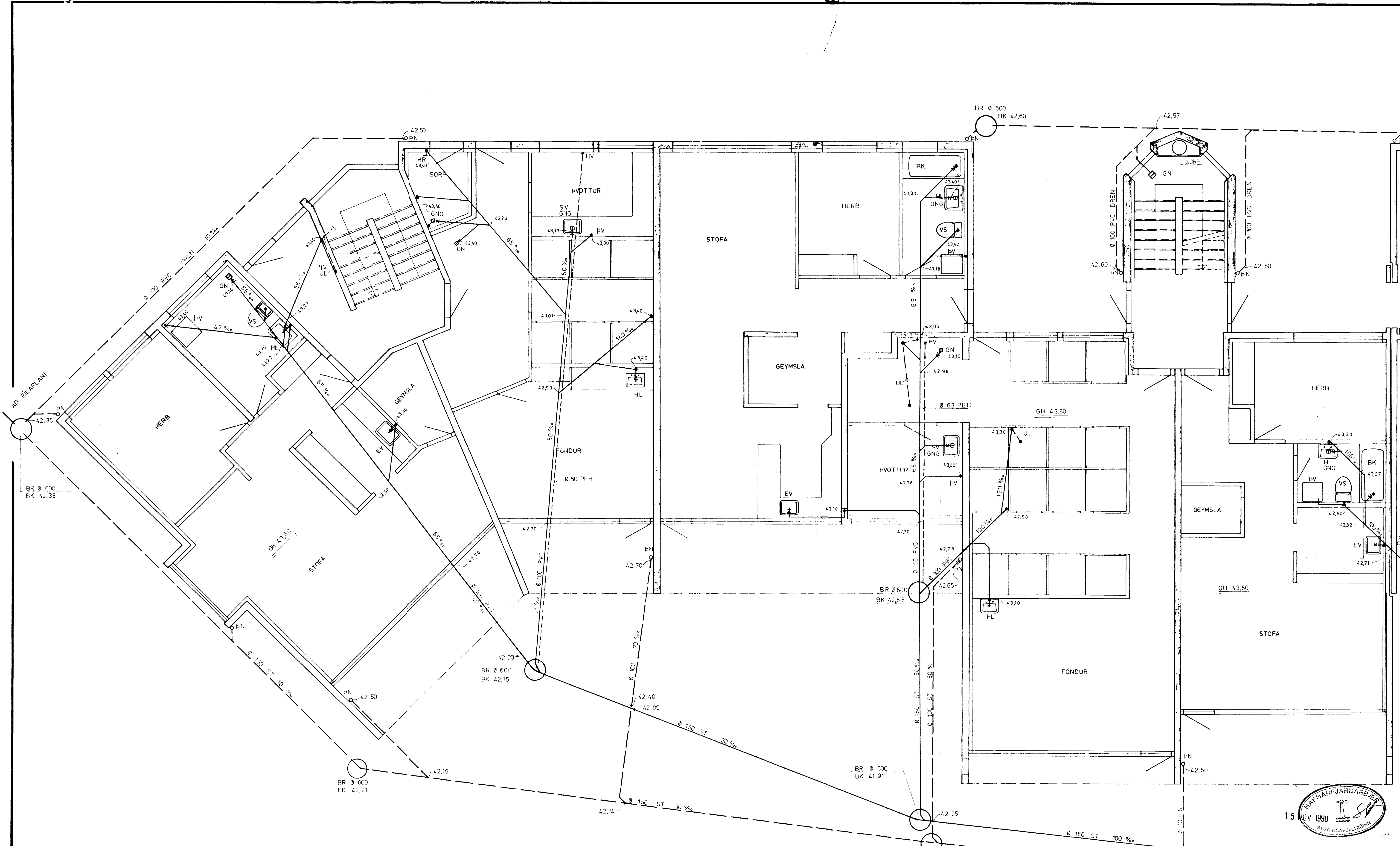
GRUNNMYND 1. HÆÐ 1:50
