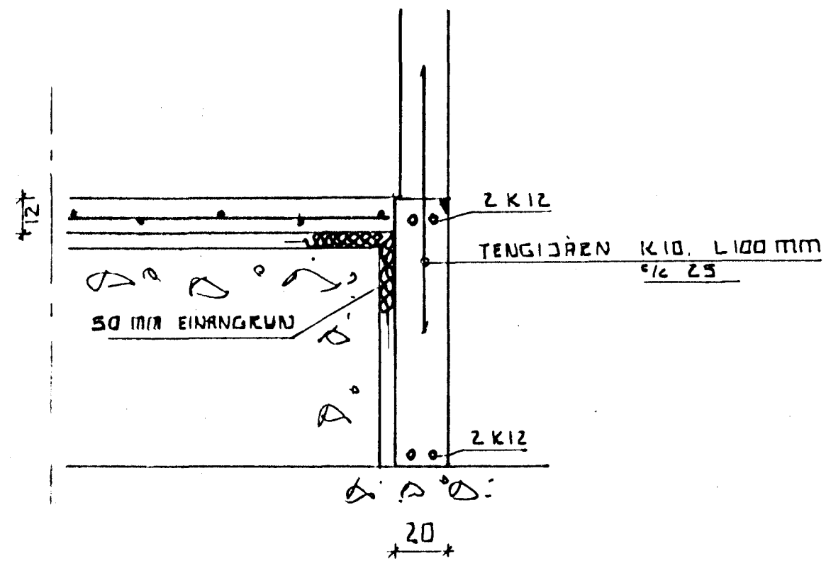
A-A 1:20
