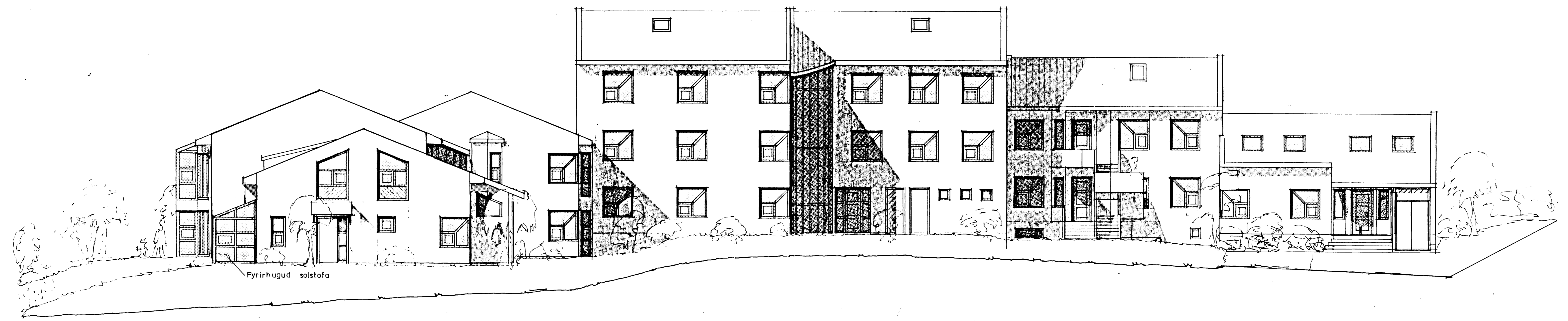
útlit austur 1:100
