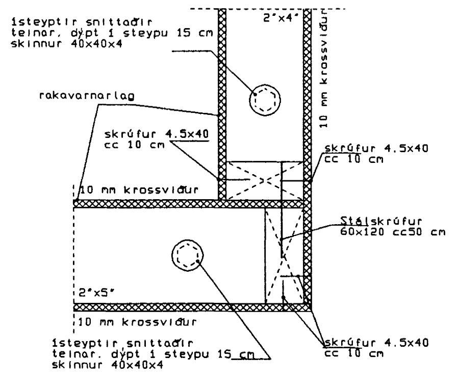
Samsetning horna lárétt sneidmynd Mkv 1:5
