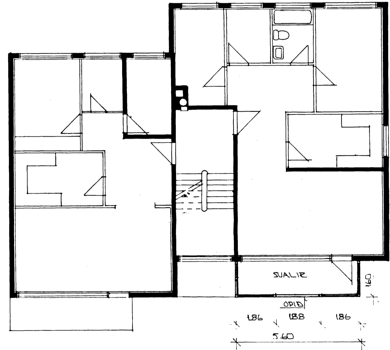
GRUNNMÝND 1. HÆÐ 1:100
