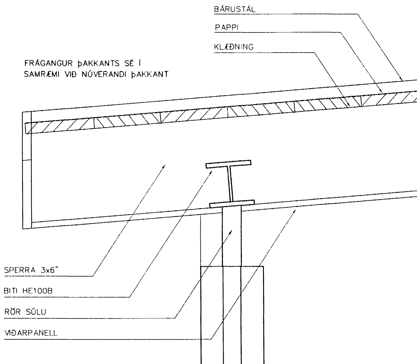
ÞAK DEILI 1:5
