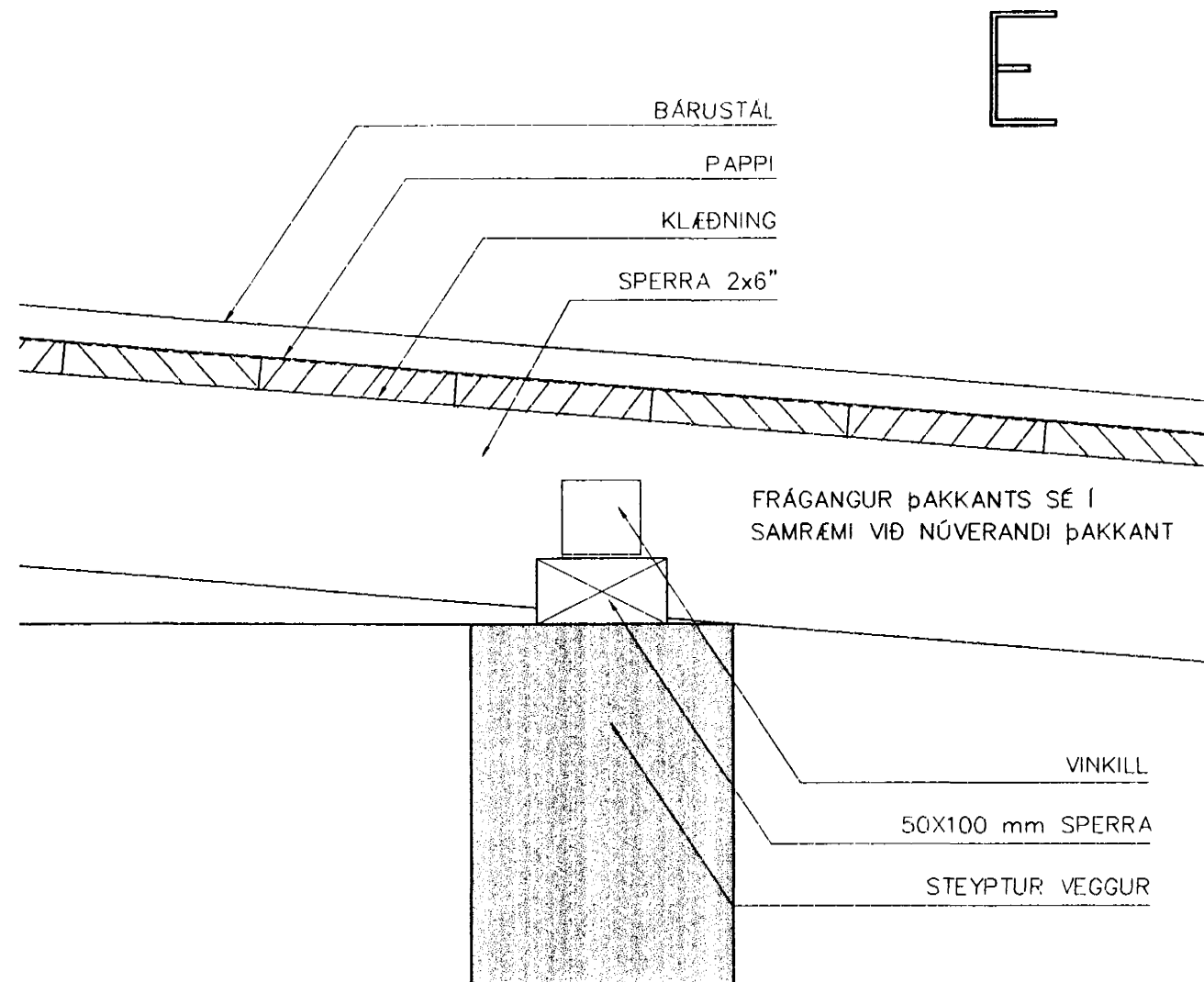
ÞAK DEILI 1:5
