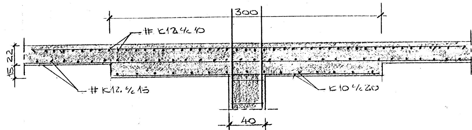
SNIP A-A 1:20
