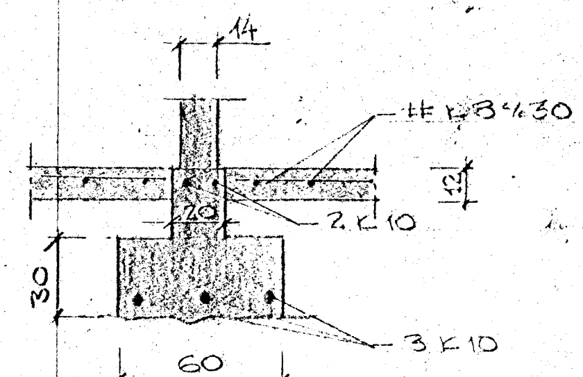
SNIP C 1:20 UNDIRSTÖÐUR UNDIR LINDUVEGI
