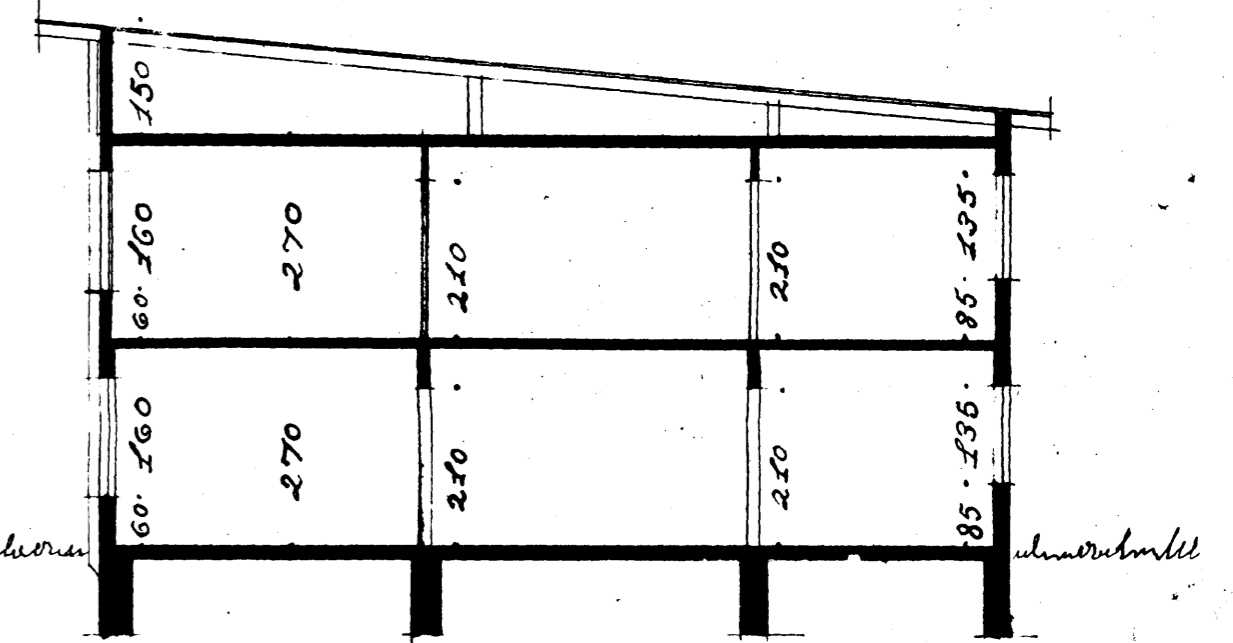
Sneiðing.
