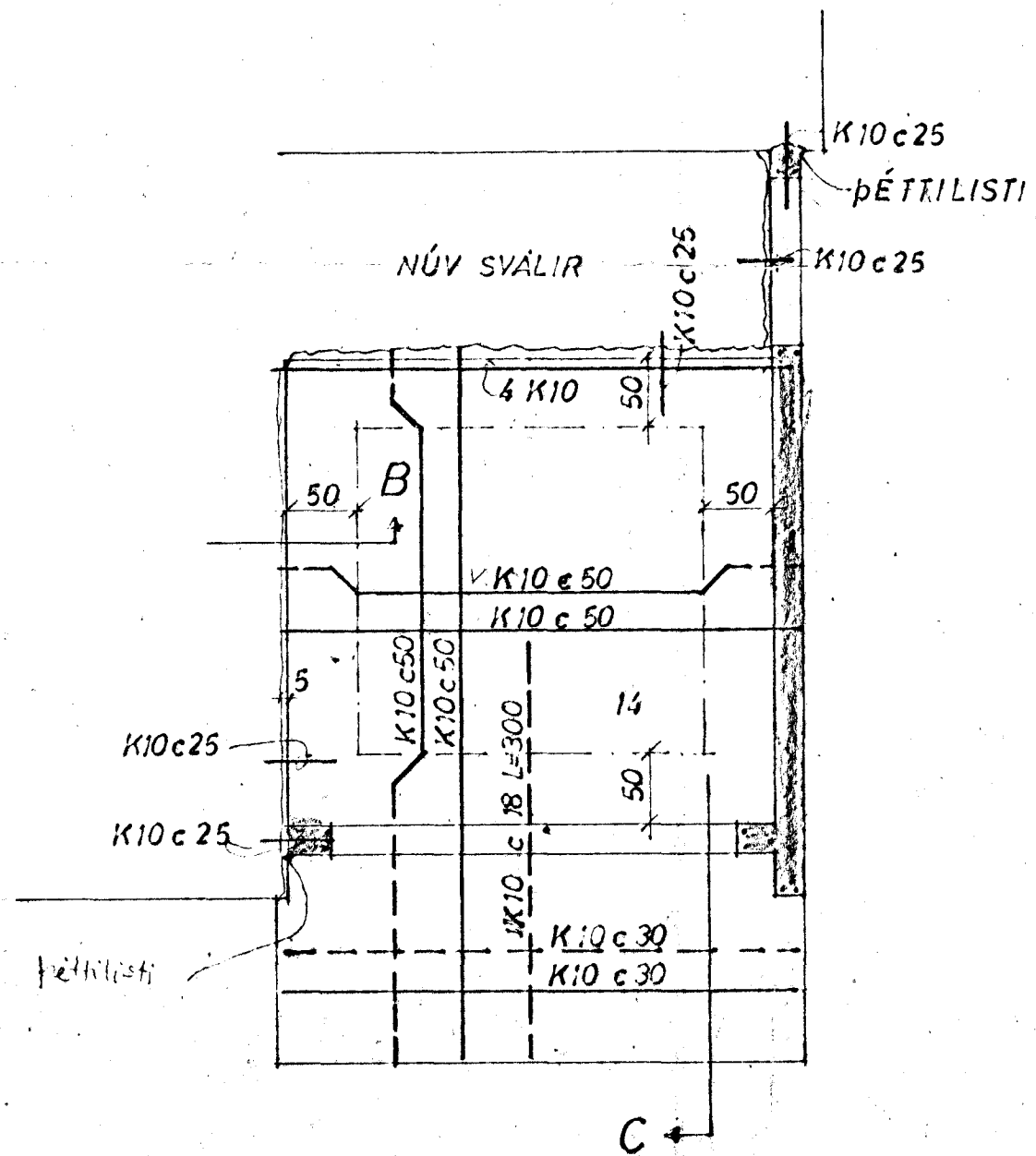
LOFT YFIR 1 OG 2. HÆÐ.
