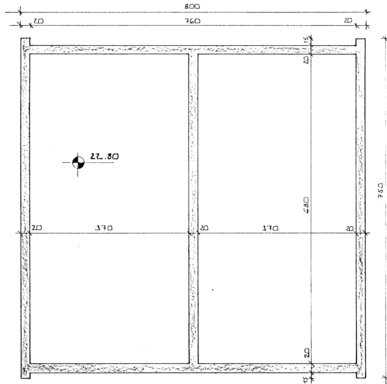
GRUNNMYND ~ 1:50 UNDIRSTÖÐUR
