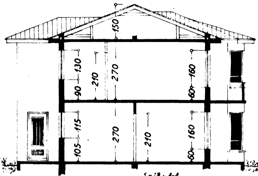
Sníð: A-A
