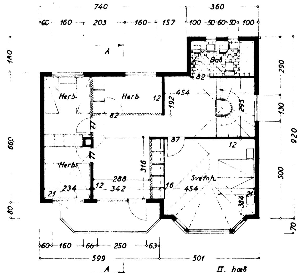
II. hæð
