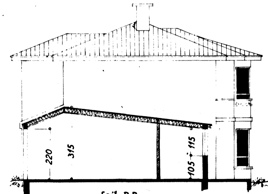
Sníð: B-B
