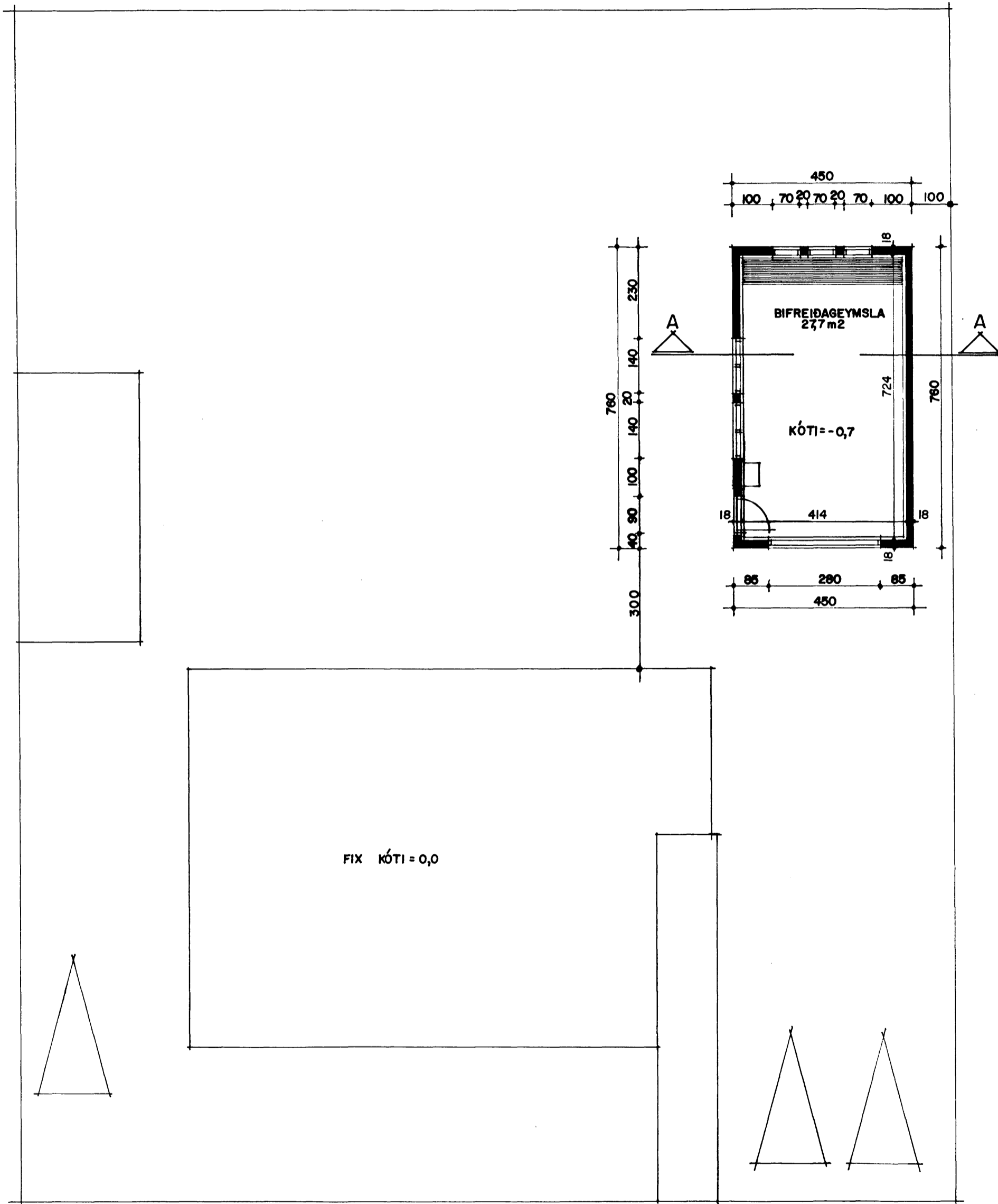
GRUNNMYND I HÆÐ MKV. 1:100
