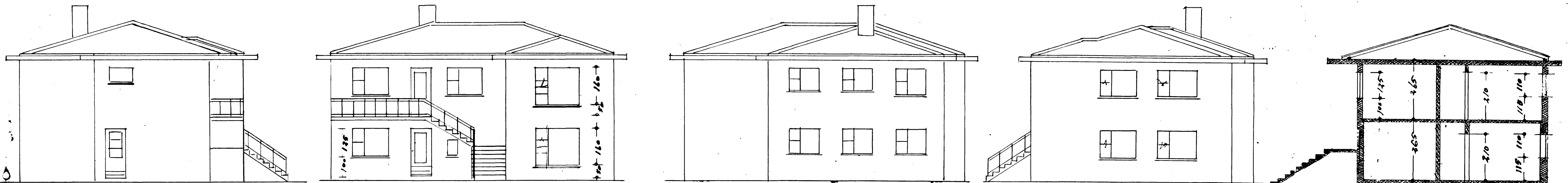
NORDVESTUR.
