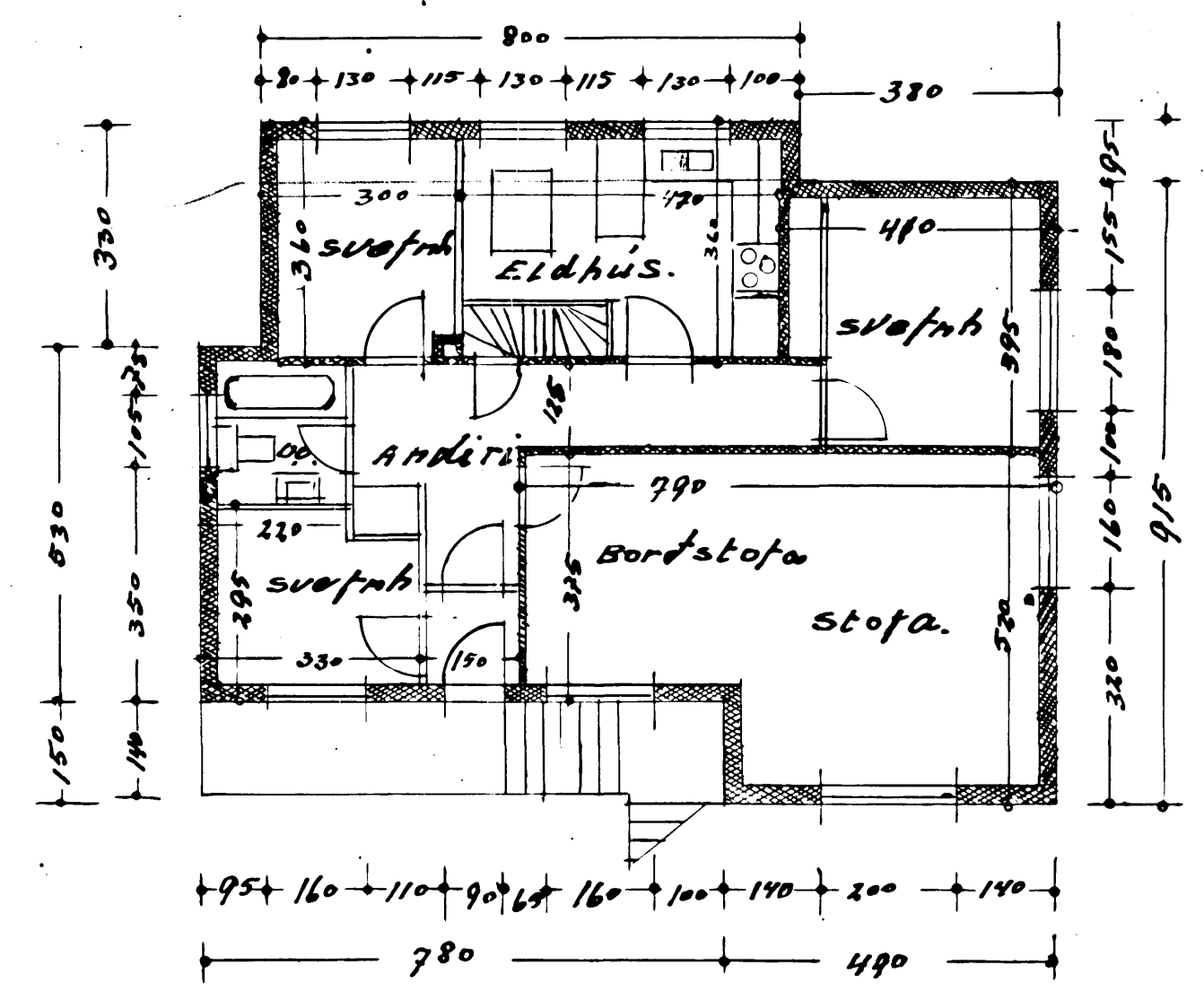
1 HÆÐ.
