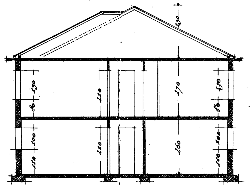
a-a
