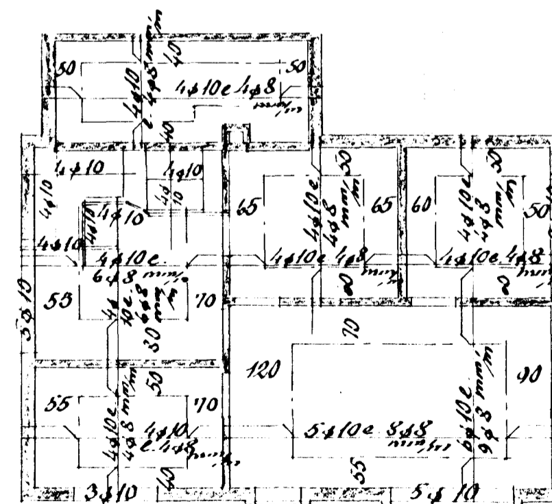
Loft yfir kjallara 1:100
