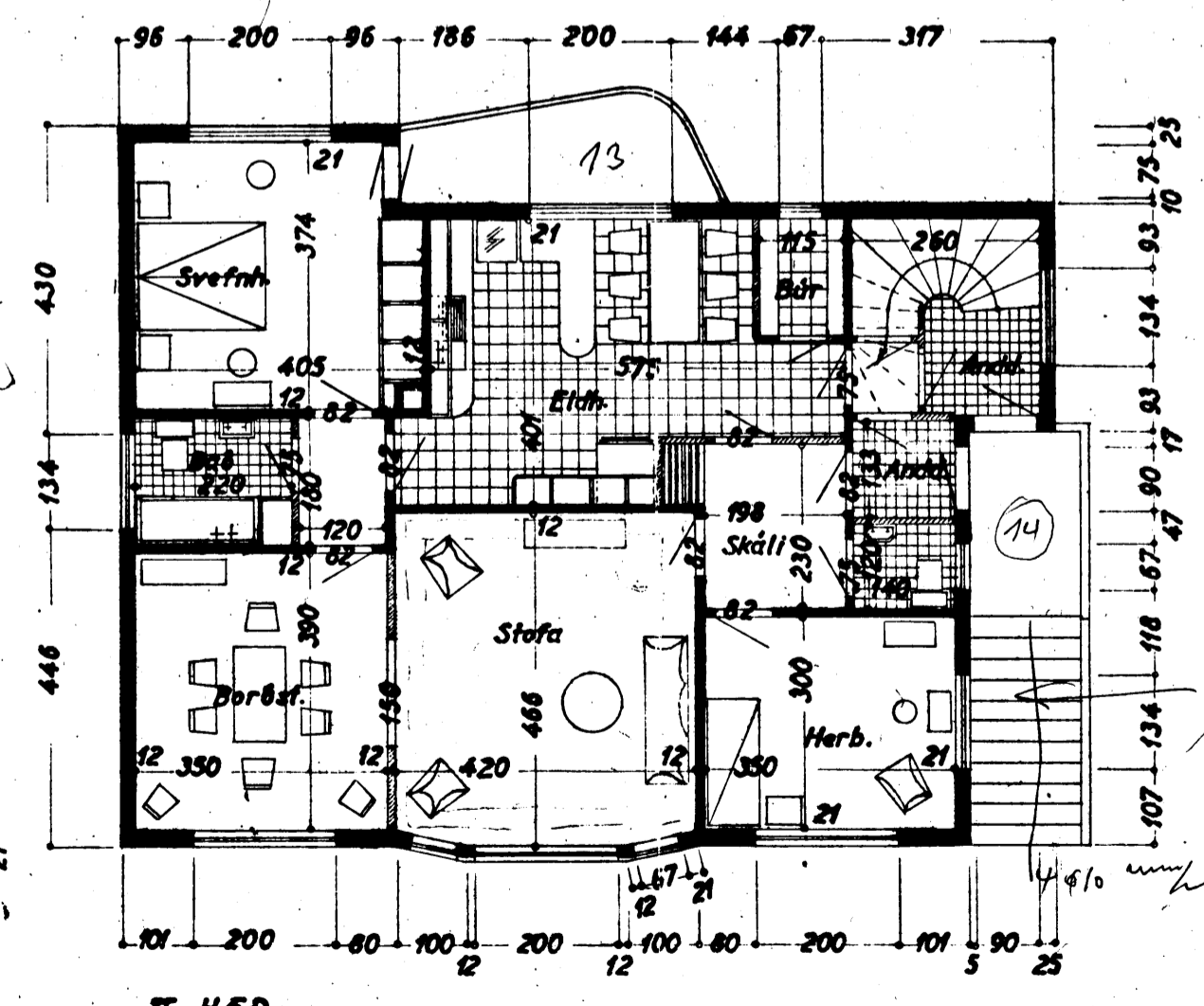
II. HÆÐ
