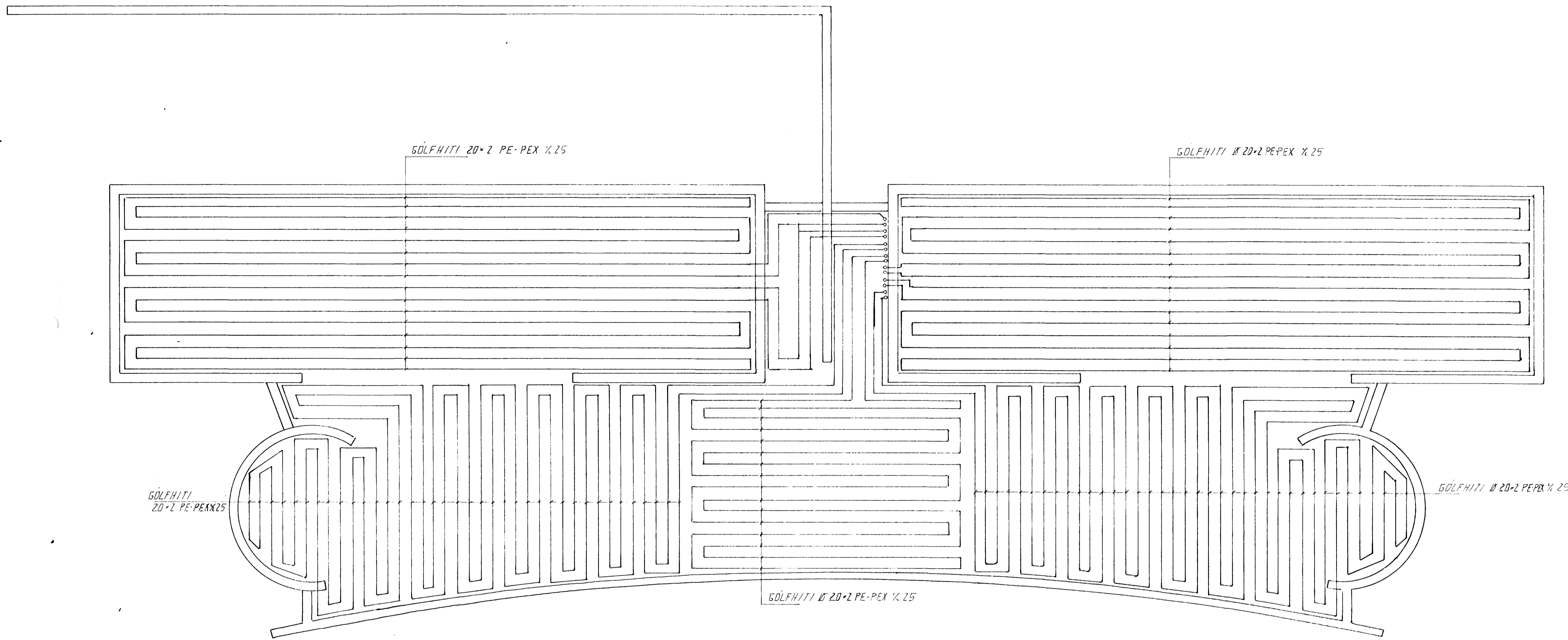
GRUNNMUND GOLFHTI 1:50
