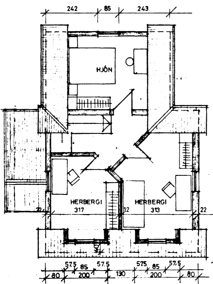
RIS 1:100
