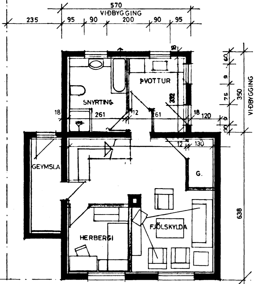
KJALLARI 1:100
