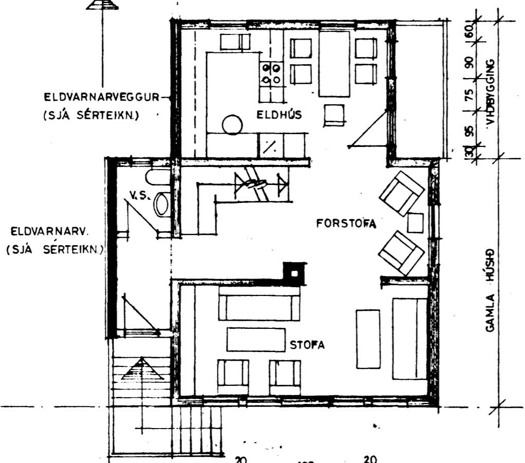
HÆÐ 1:100
