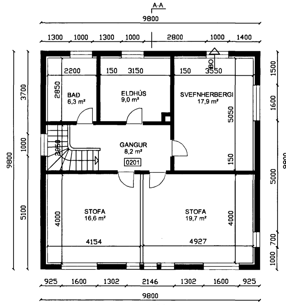
GRUNNMYND AF 2. HÆÐ
