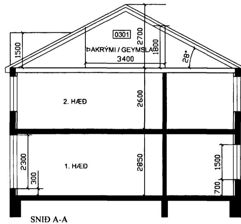
SNÍÐ A-A
