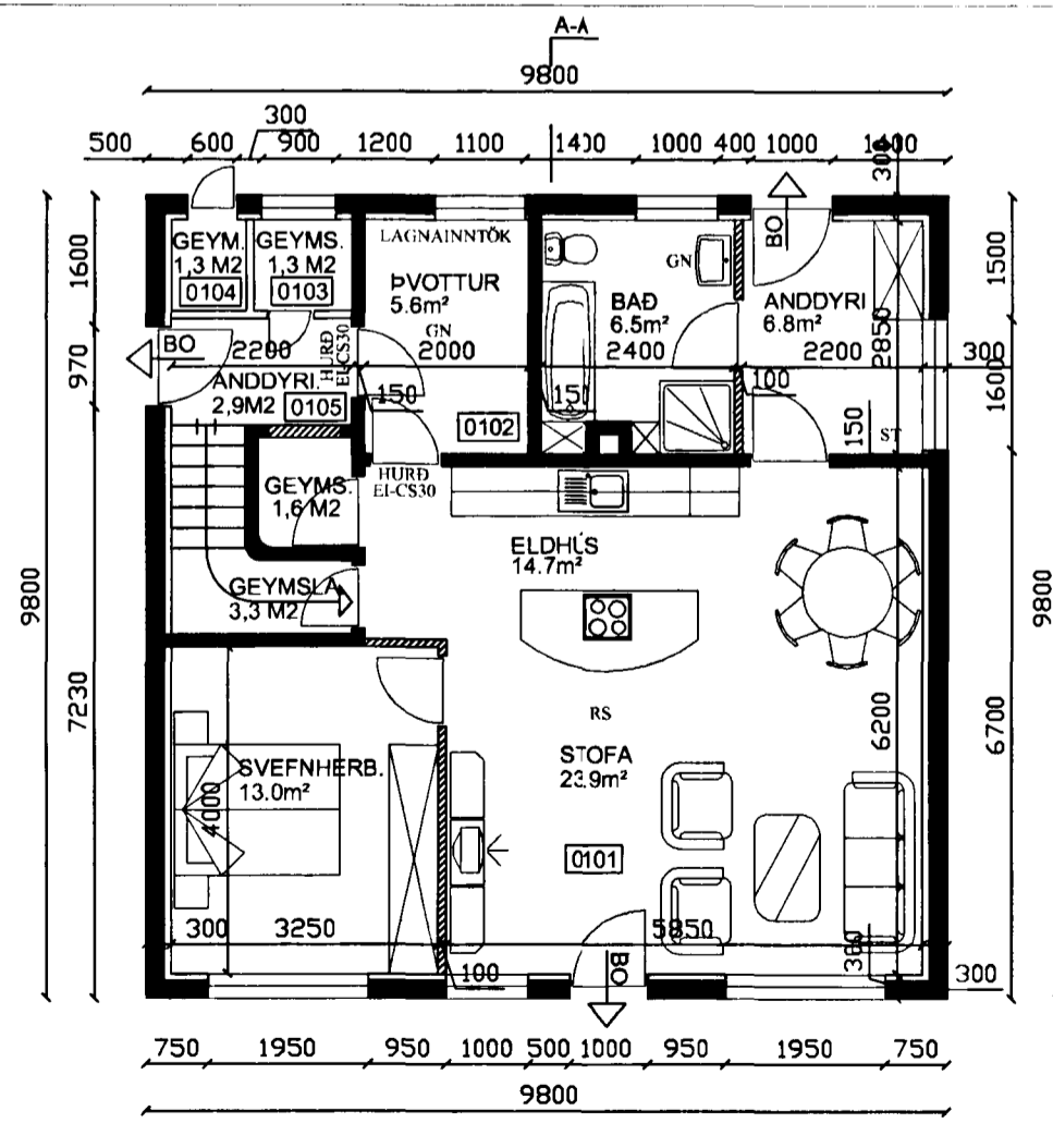
GRUNNMYND AF 1. HÆÐ
