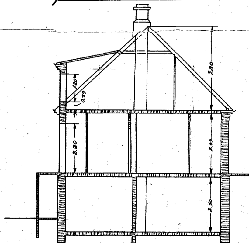
Þverskurður A.A.
