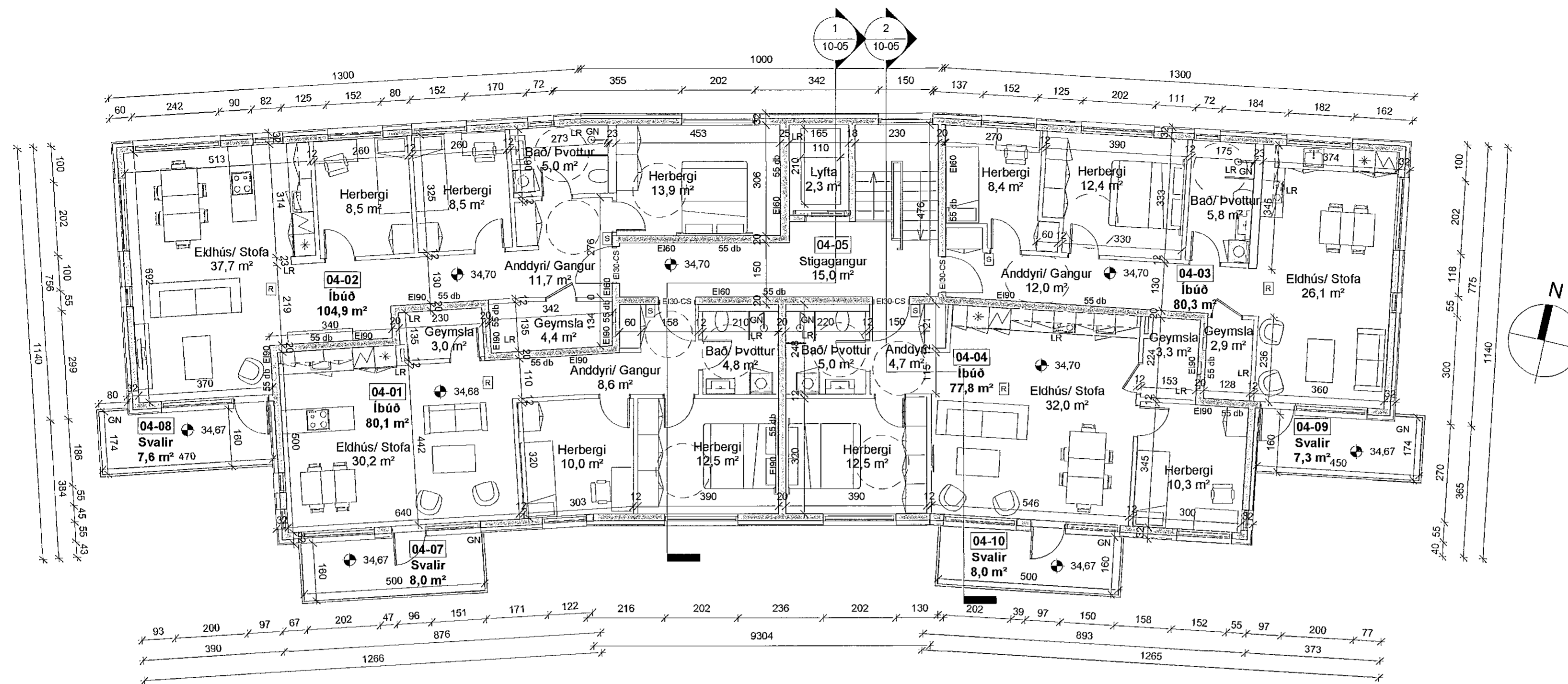
4. hæð Mhl. 02 1 : 100
