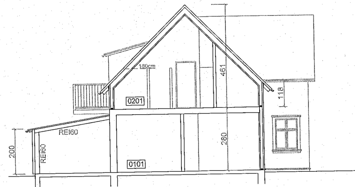
Sneiðing aa 1:100
