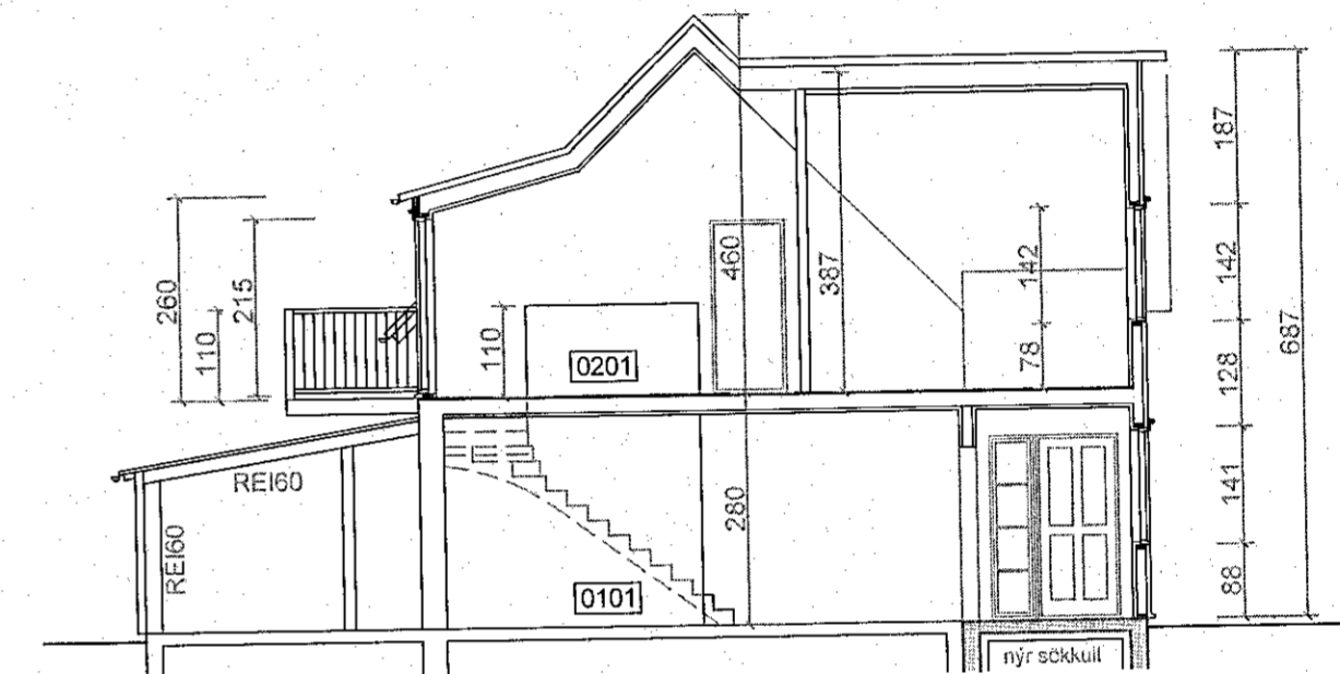
Sneiðing bb 1:100
