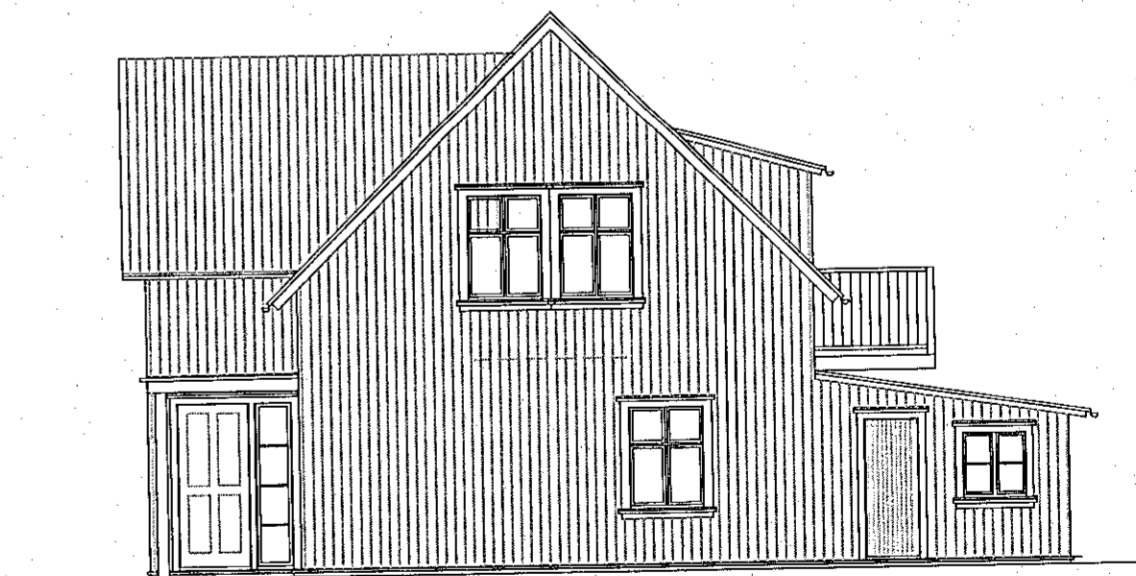
Útlit vestur 1:100
