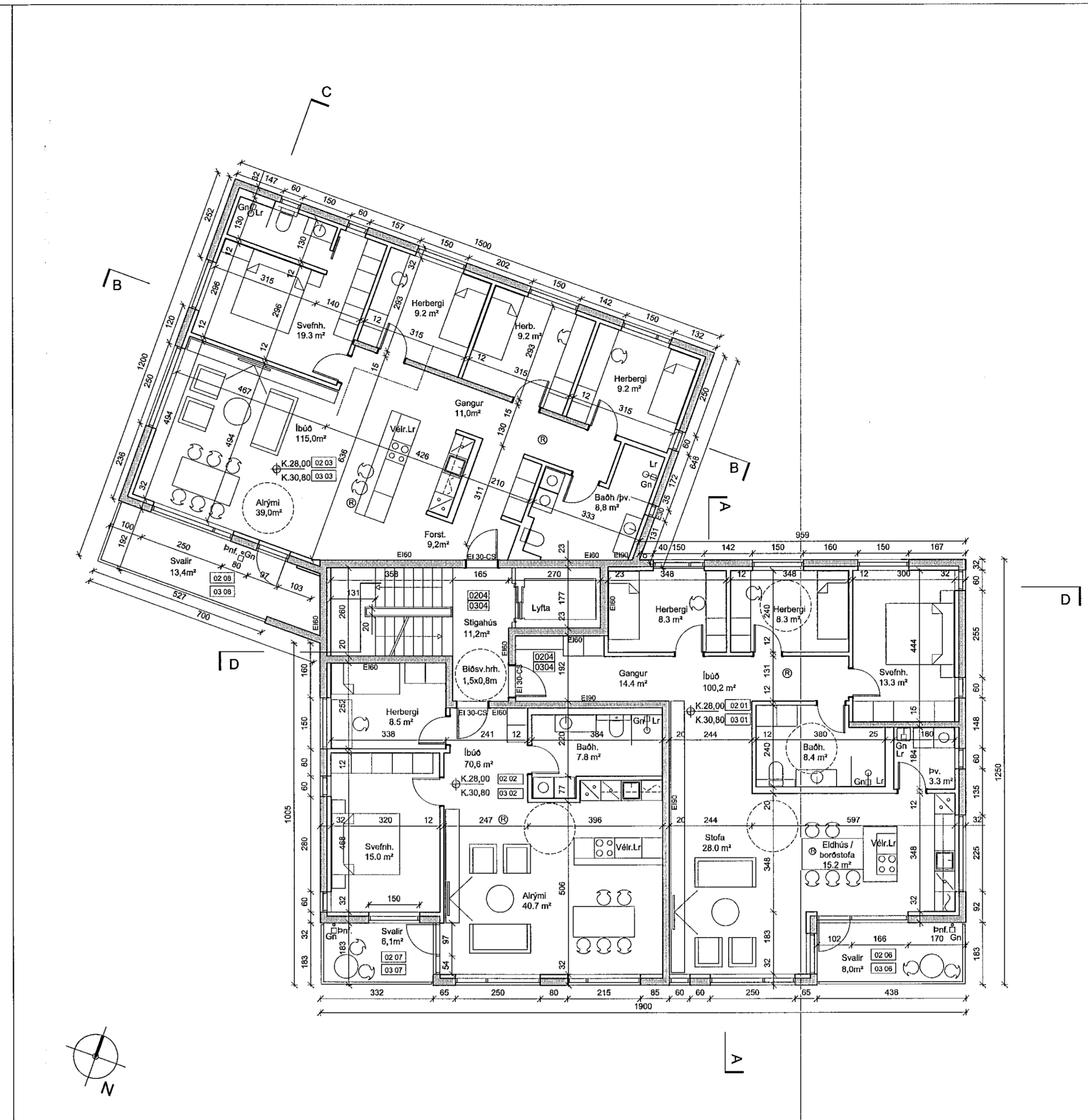
GRUNNMYND 2-3 HÆÐ
