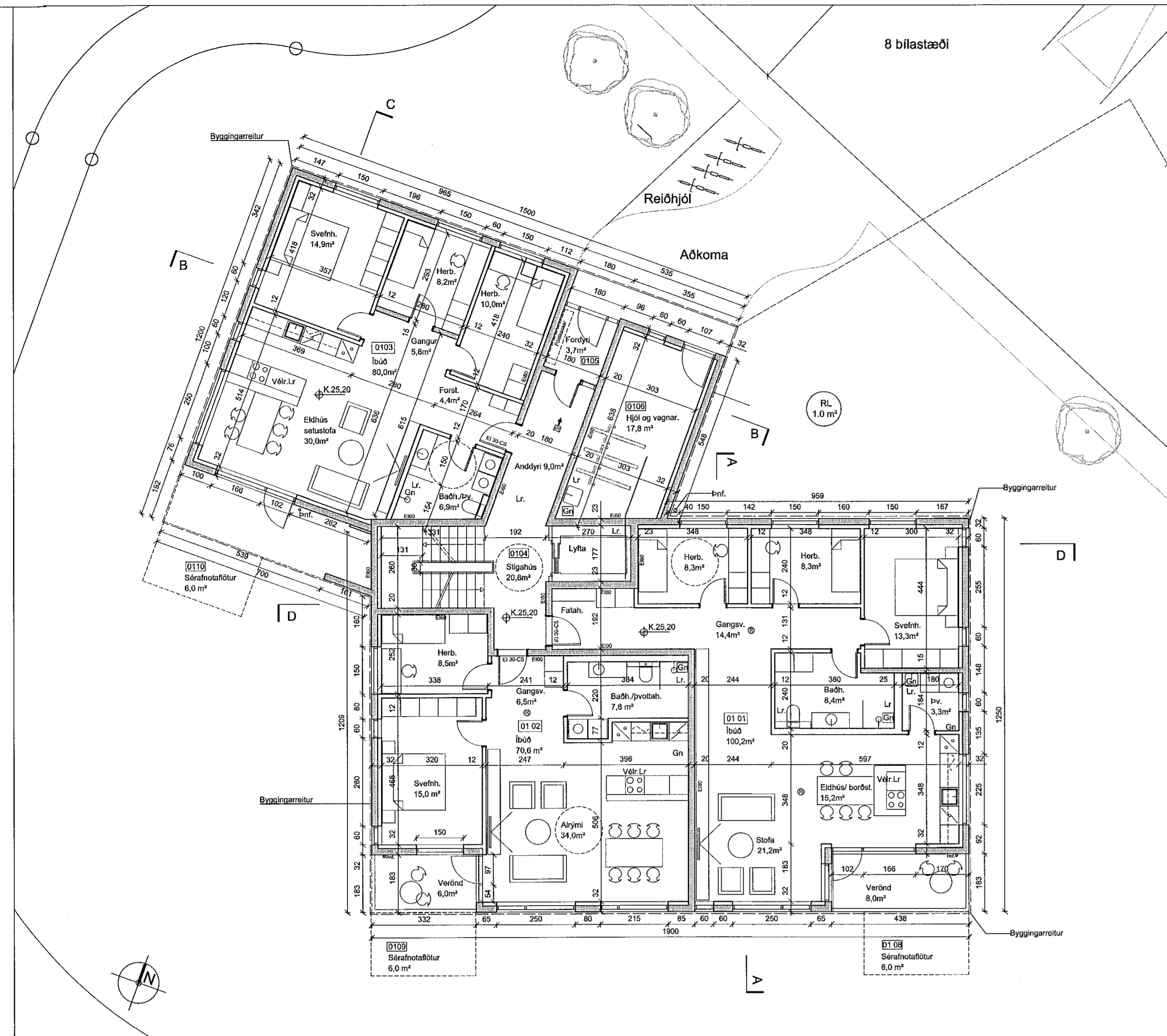
GRUNNMYND 1.HÆÐ
