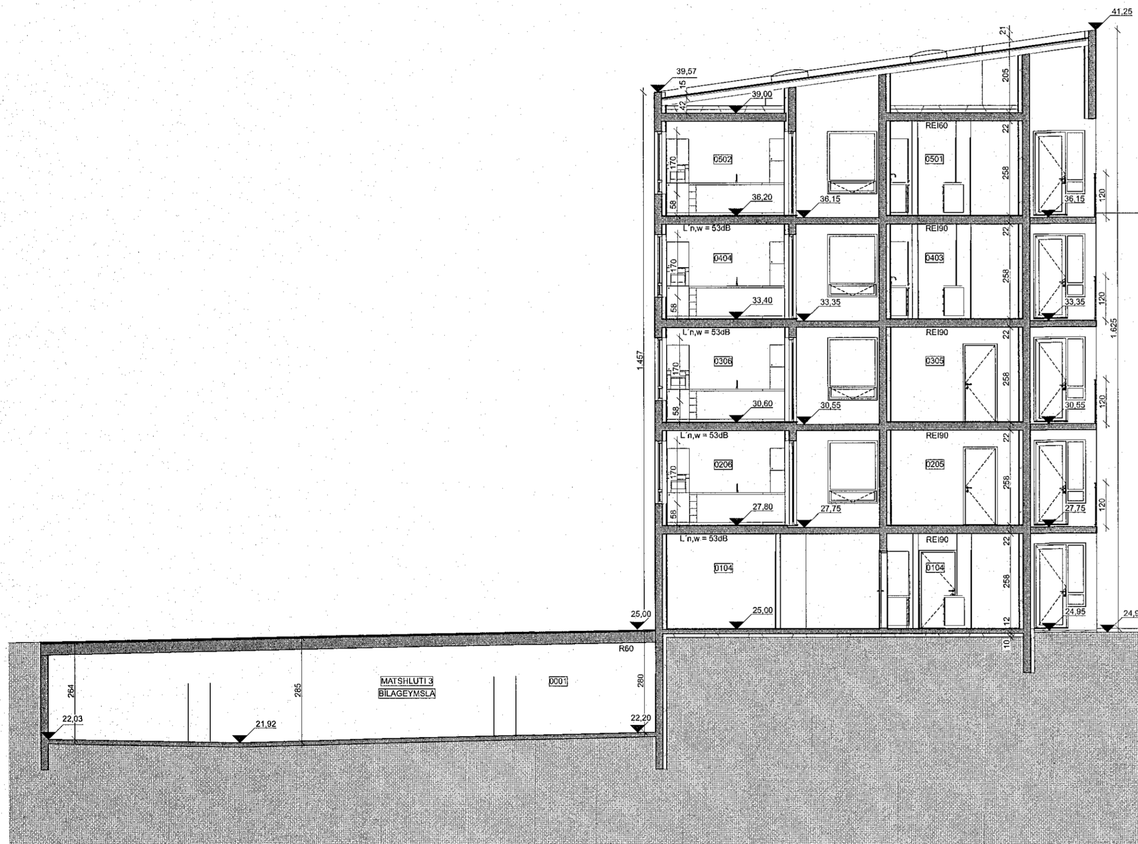
A-A
