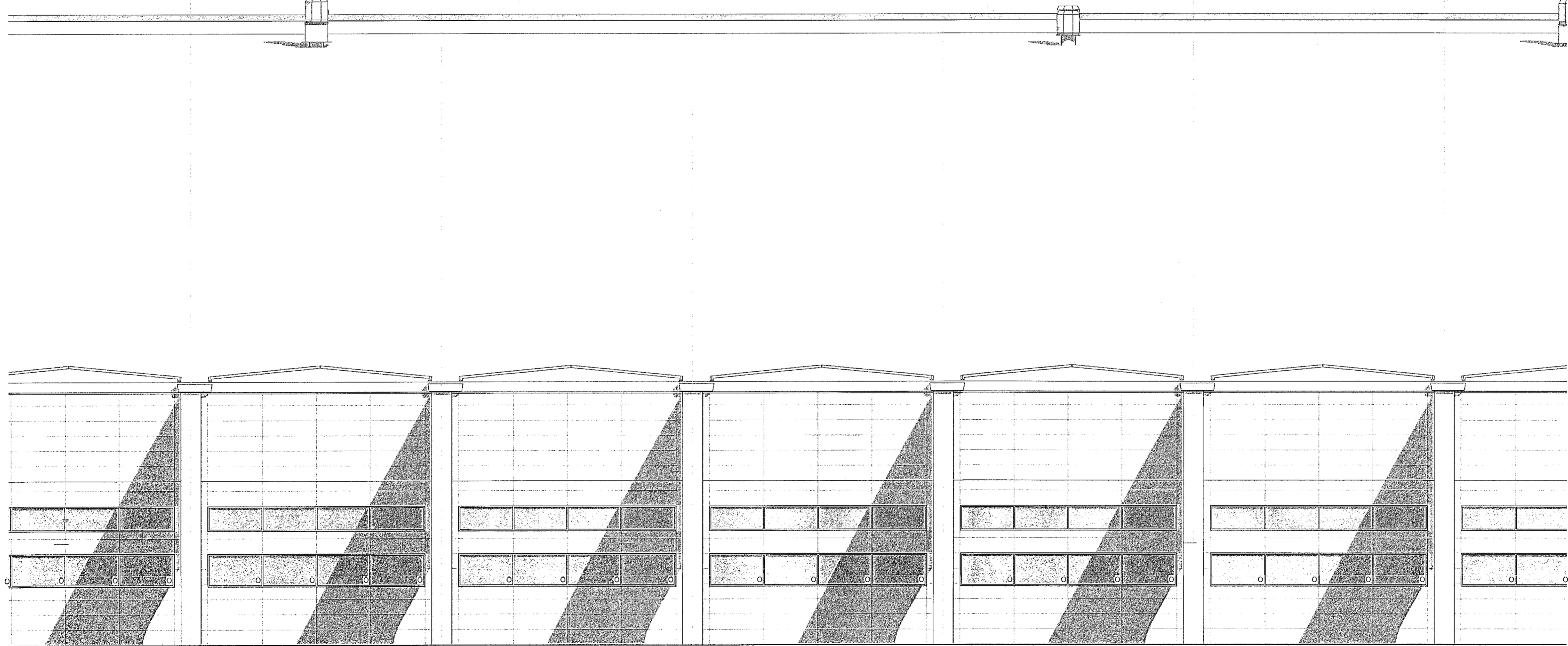
2 Vestur - Hluti 2 1 : 100
