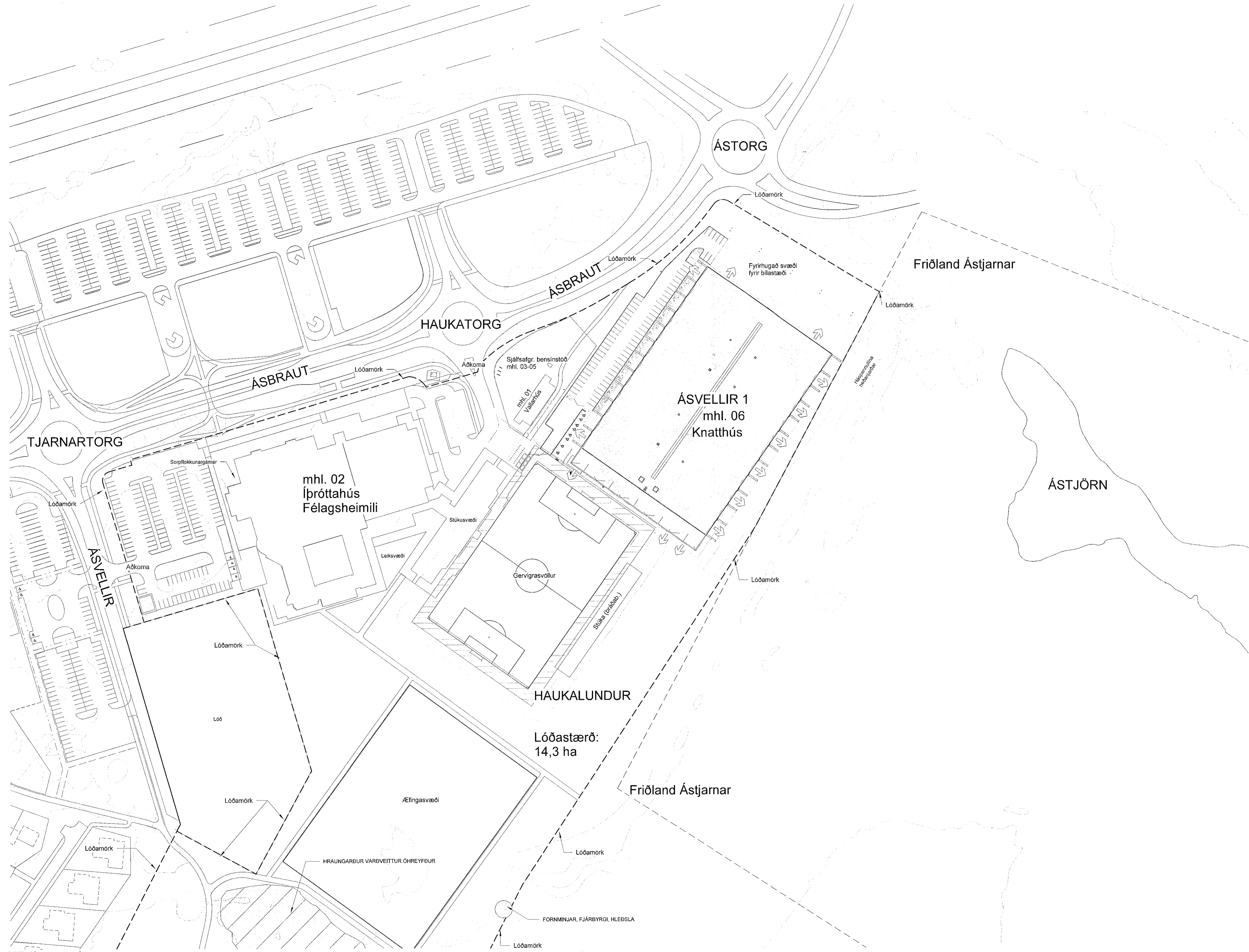
1 Yfirlitsmynd 1 : 1000
