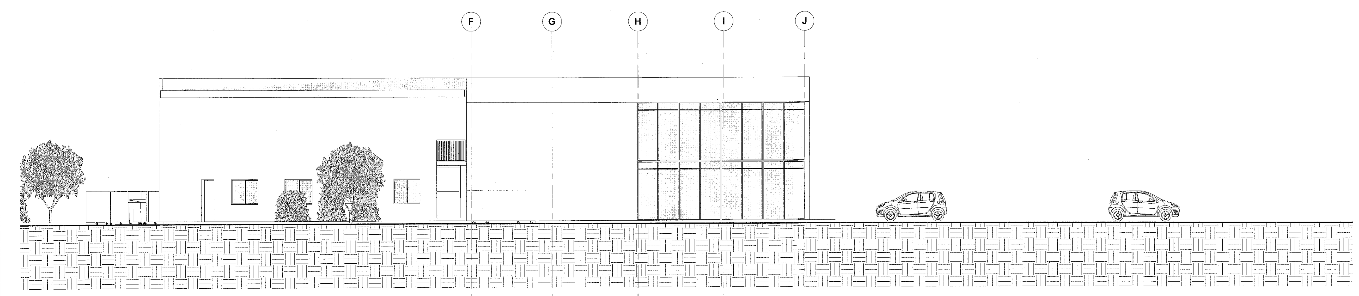
NORÐAUSTUR 1 : 100
