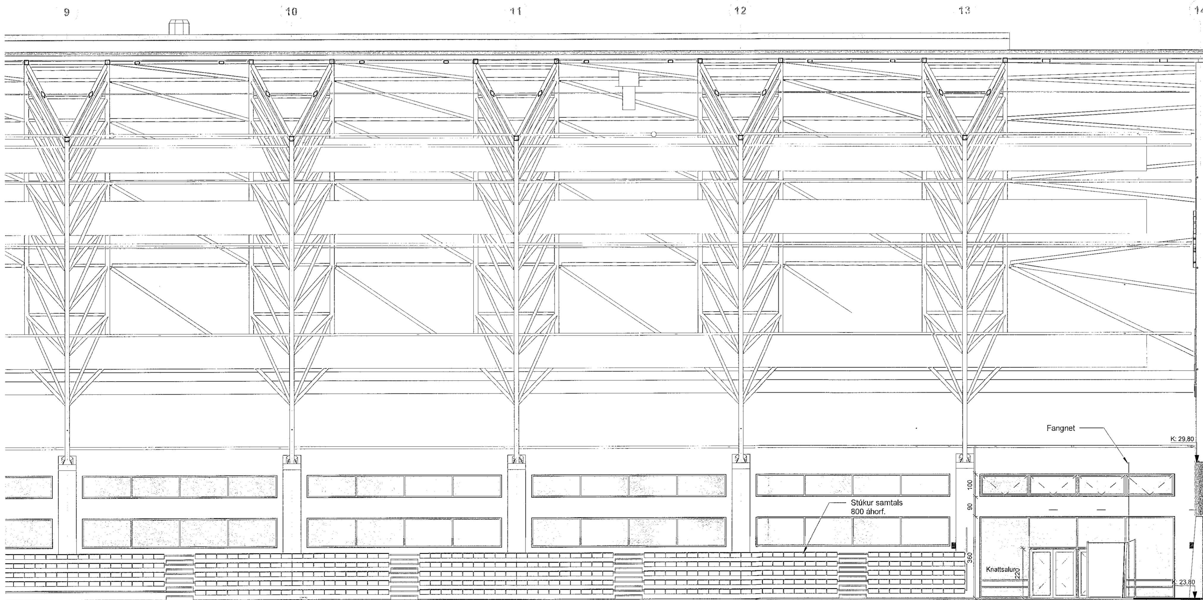
2 Sneiðing C-C - Hluti 3 1:100
