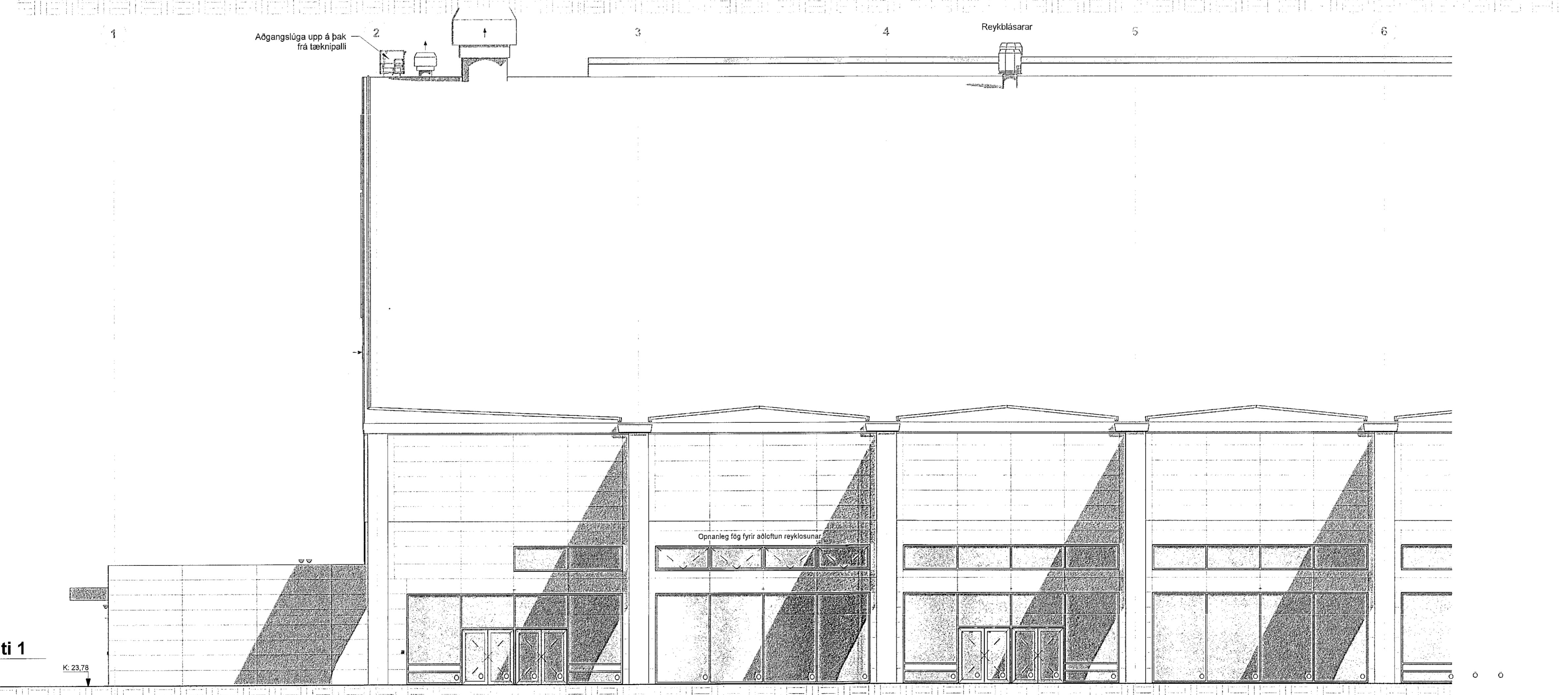
1 Vestur - Hluti 3 1 : 100
