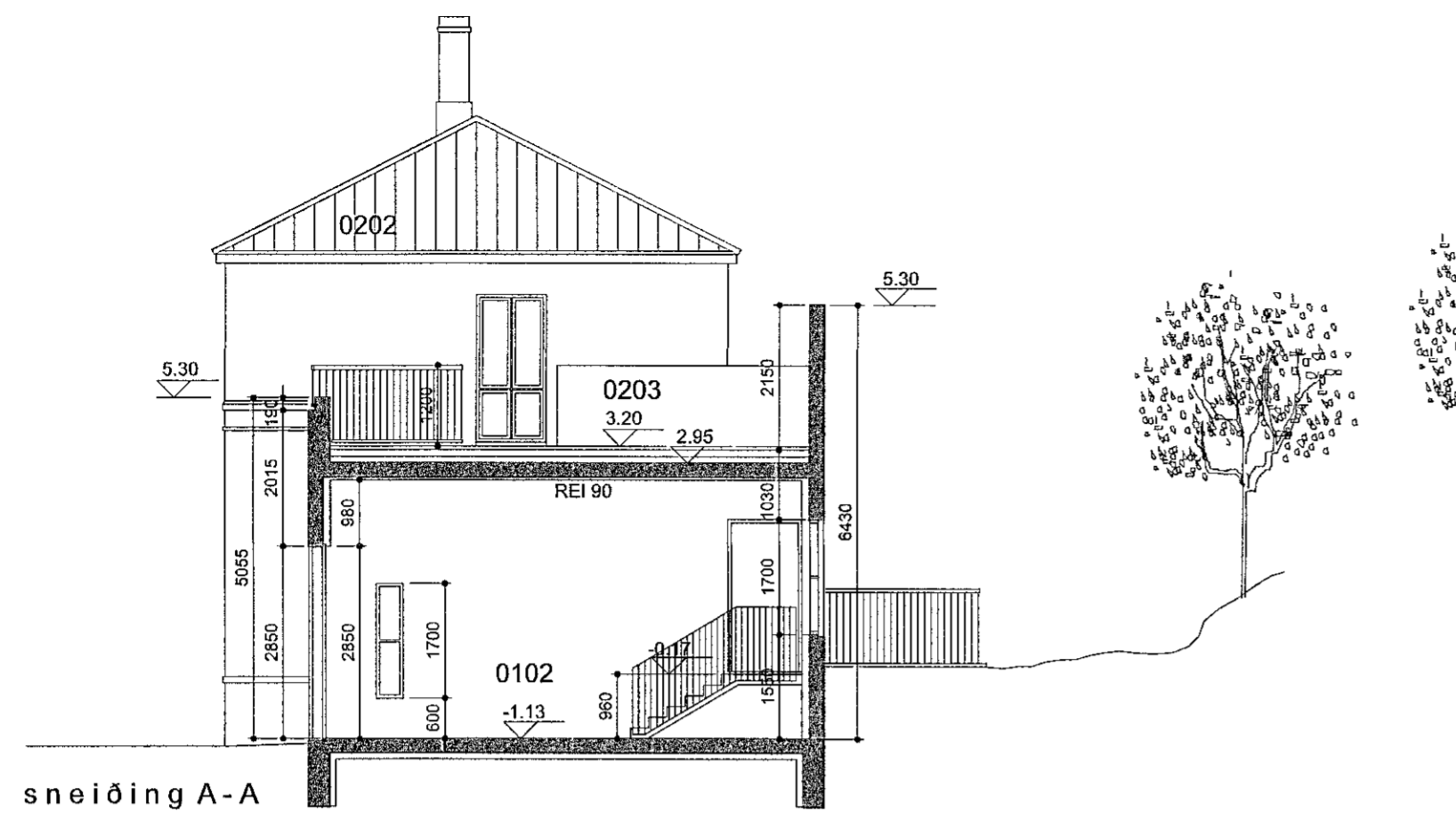
sneiðing A-A
