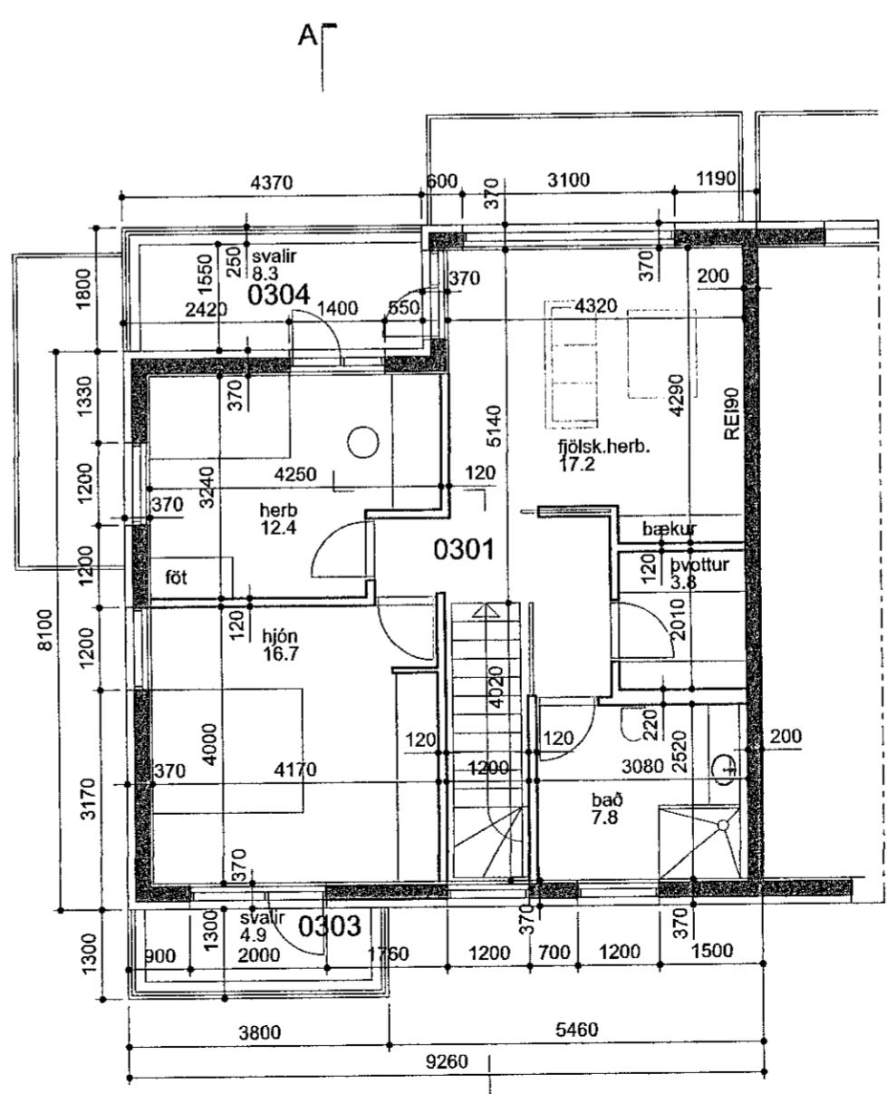
grunnmynd 3.hæðar
