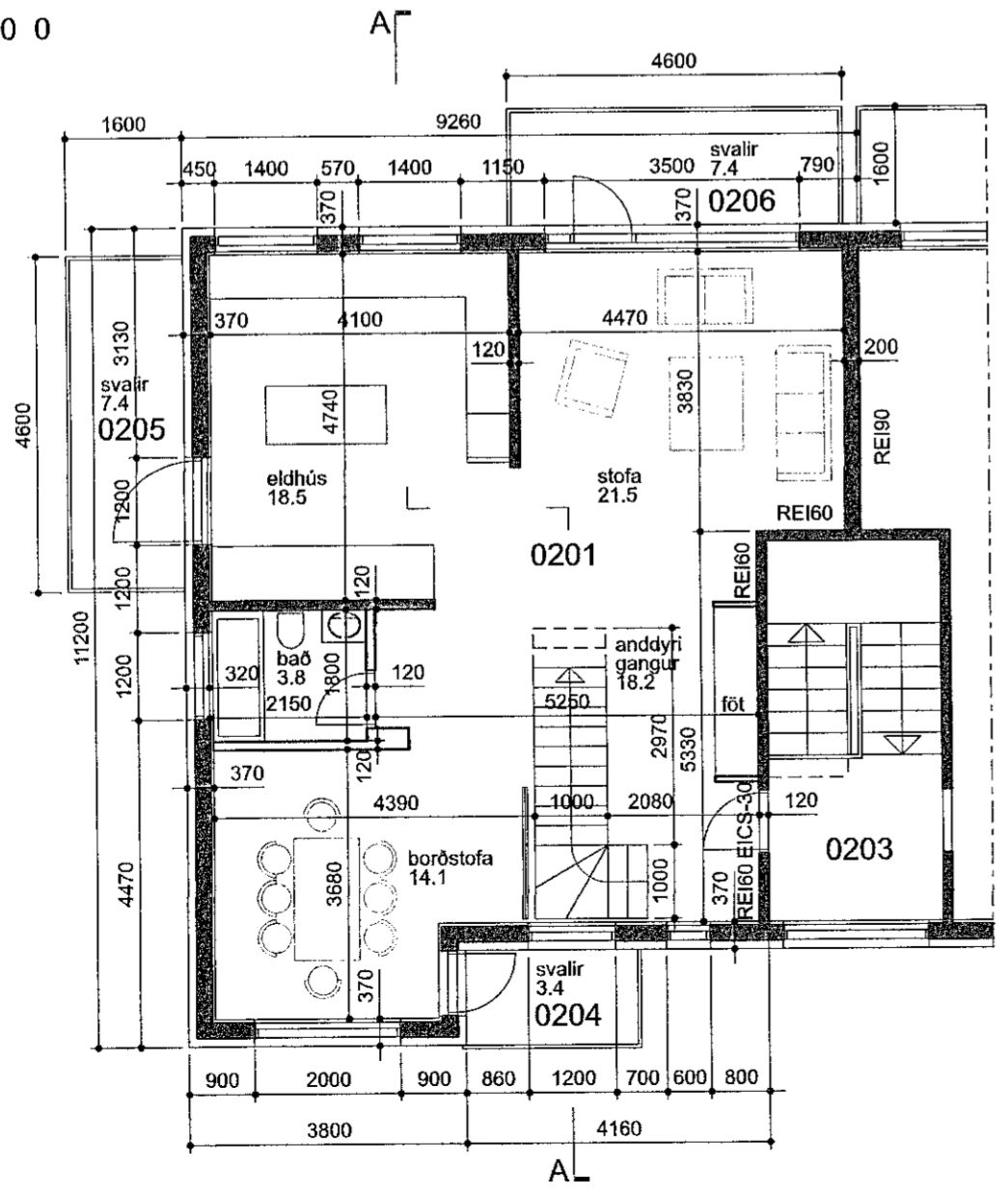
grunnmynd 2.hæðar
