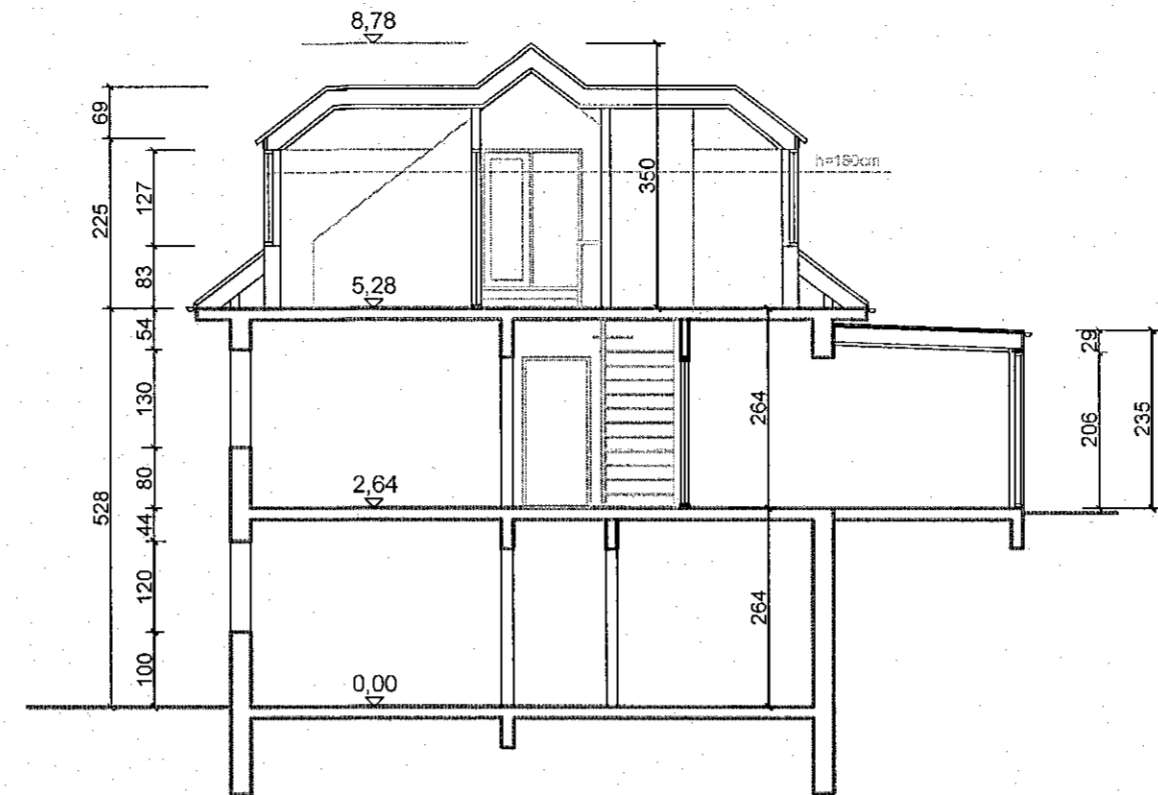
Sneiðing bb
