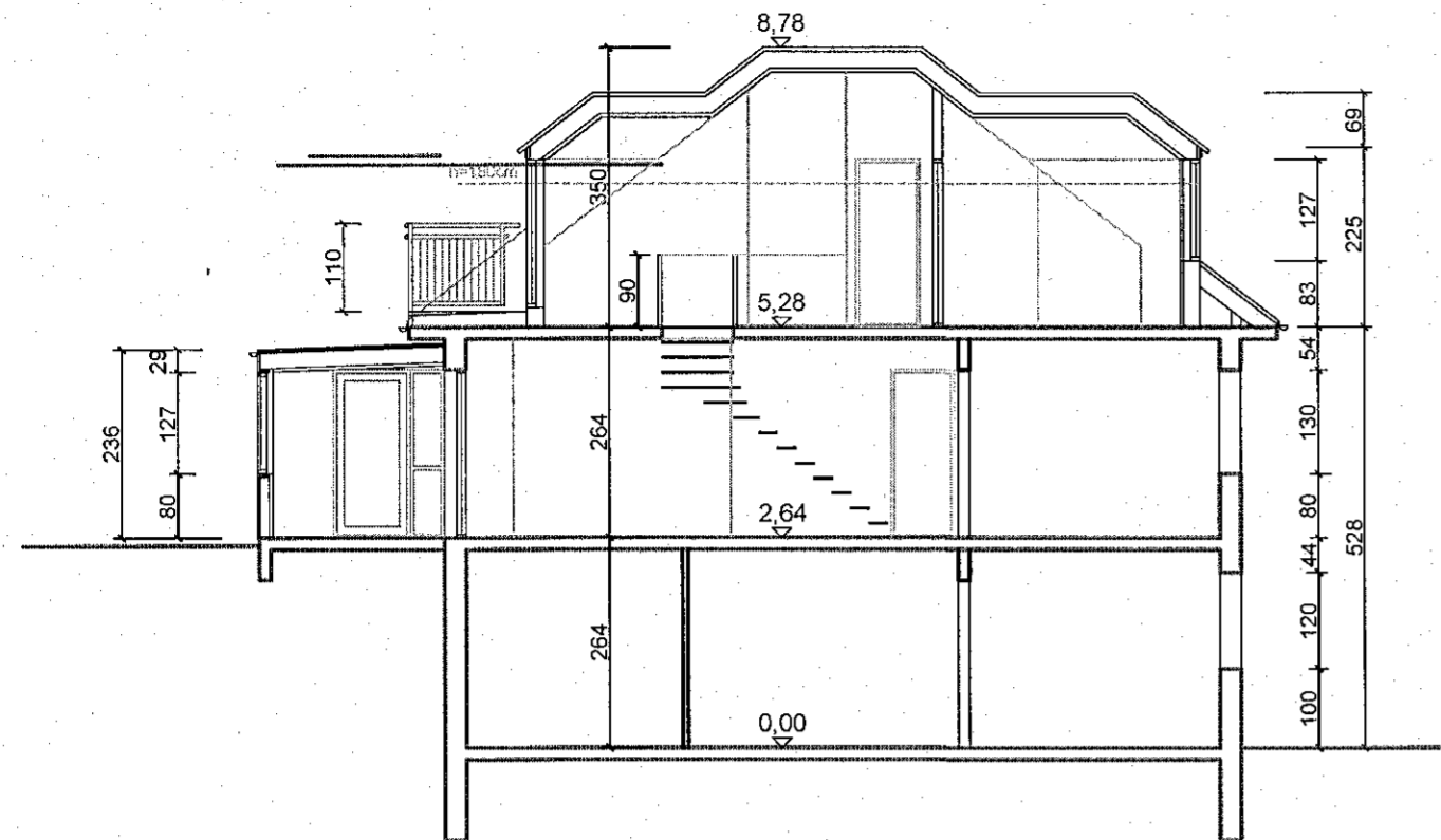
Sneiðing aa
