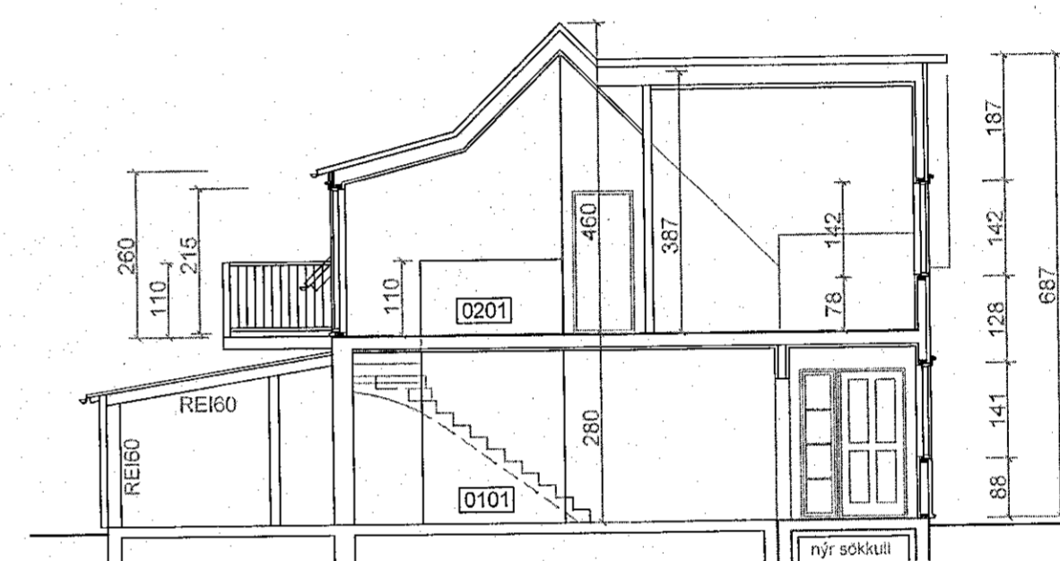
Sneiðing bb 1:100
