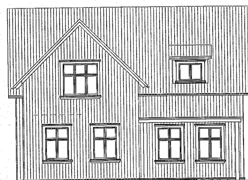
Útlit suður 1:100
