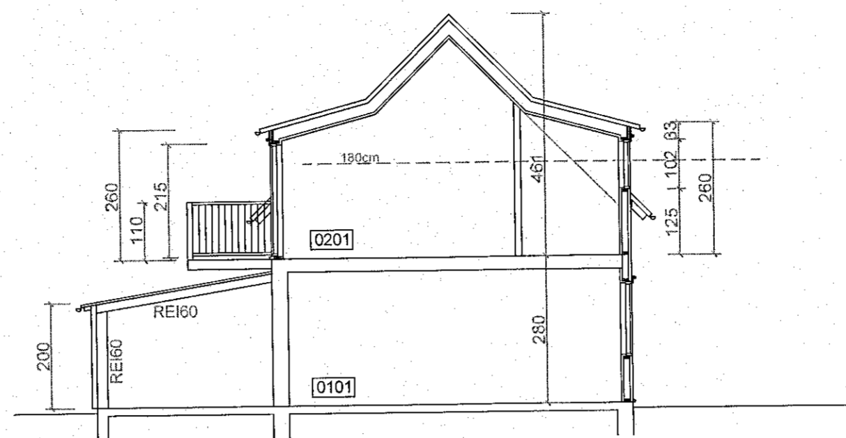
Sneiðing dd 1:100
