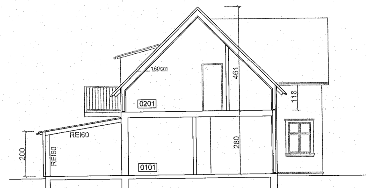
Sneiðing aa 1:100
