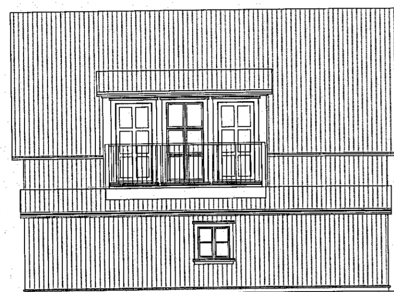
Útlit norður 1:100
