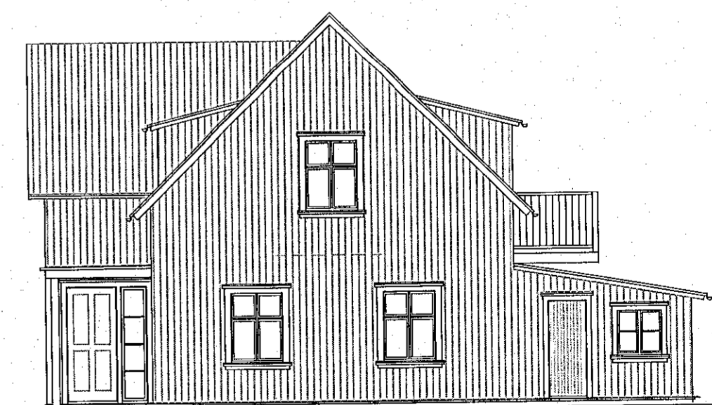
Útlit vestur 1:100
