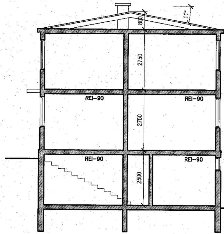
Sneiðing AA mkv. 1:100
