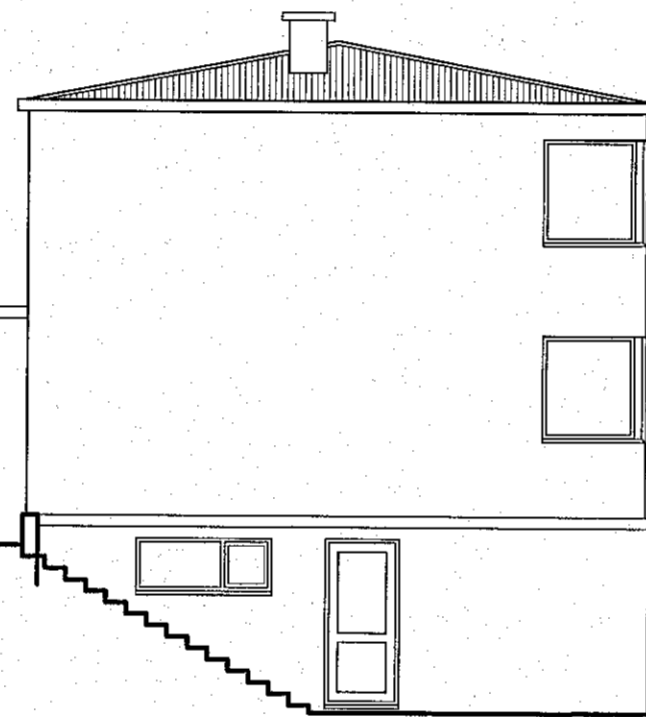
Ásýnd norður mkv. 1:100
