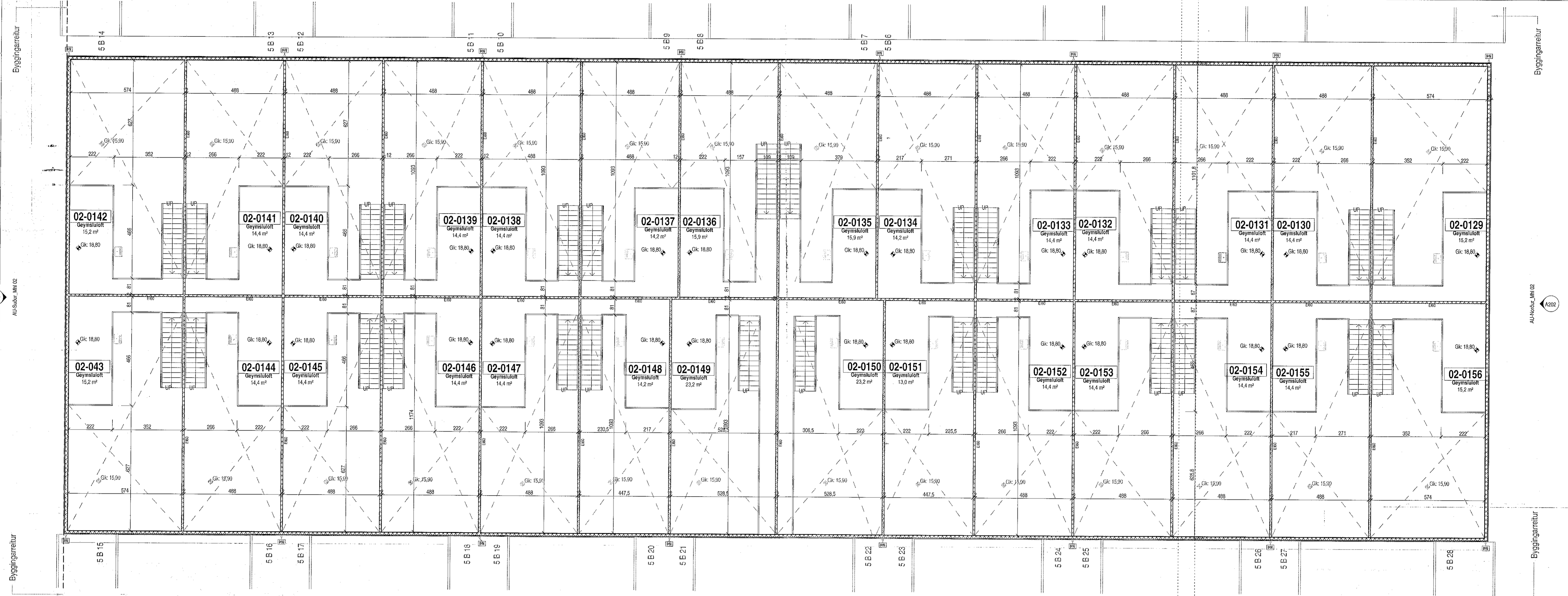
Grunnmynd geymslulofta_Mhl 02 1:100
