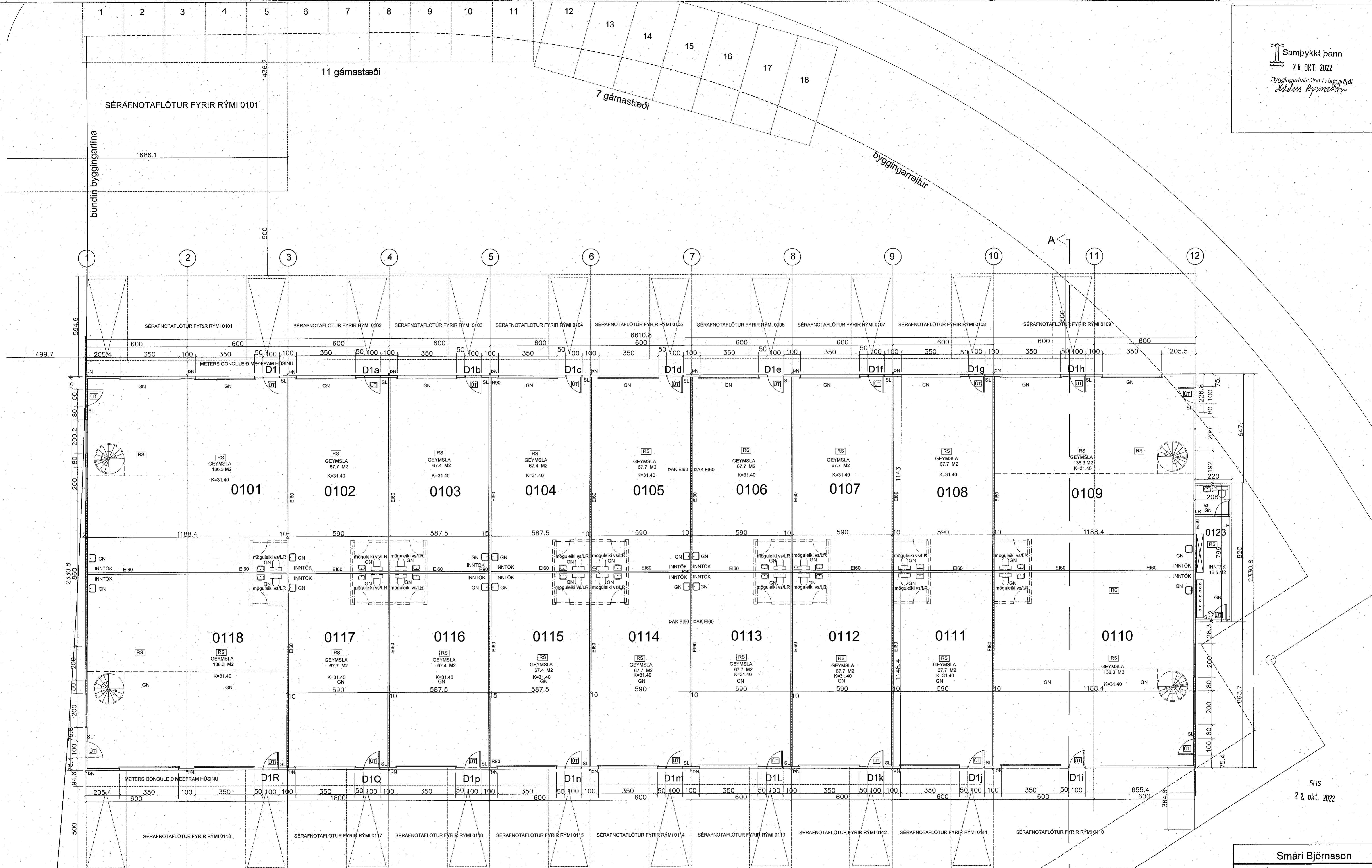
GRUNNMYND 1:100
