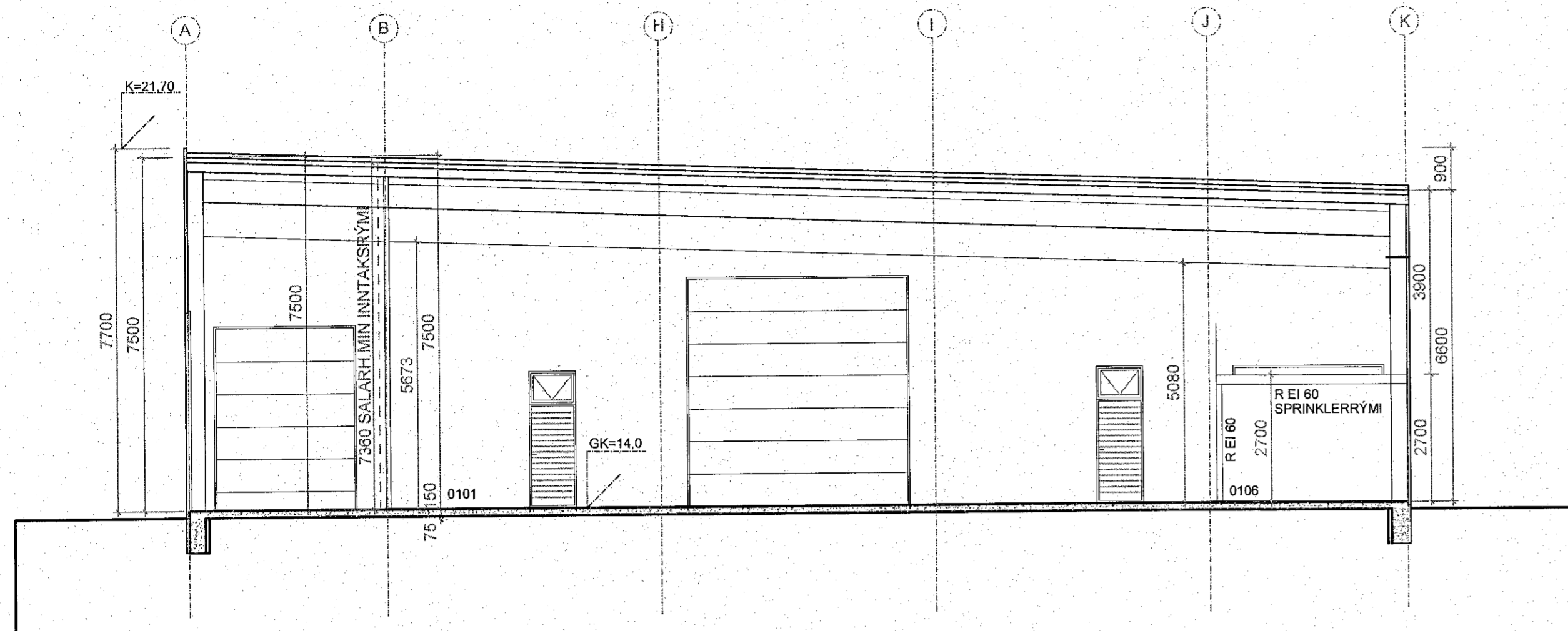
SNEIÐING B-B M1:100, NÚVERANDI HÚS
