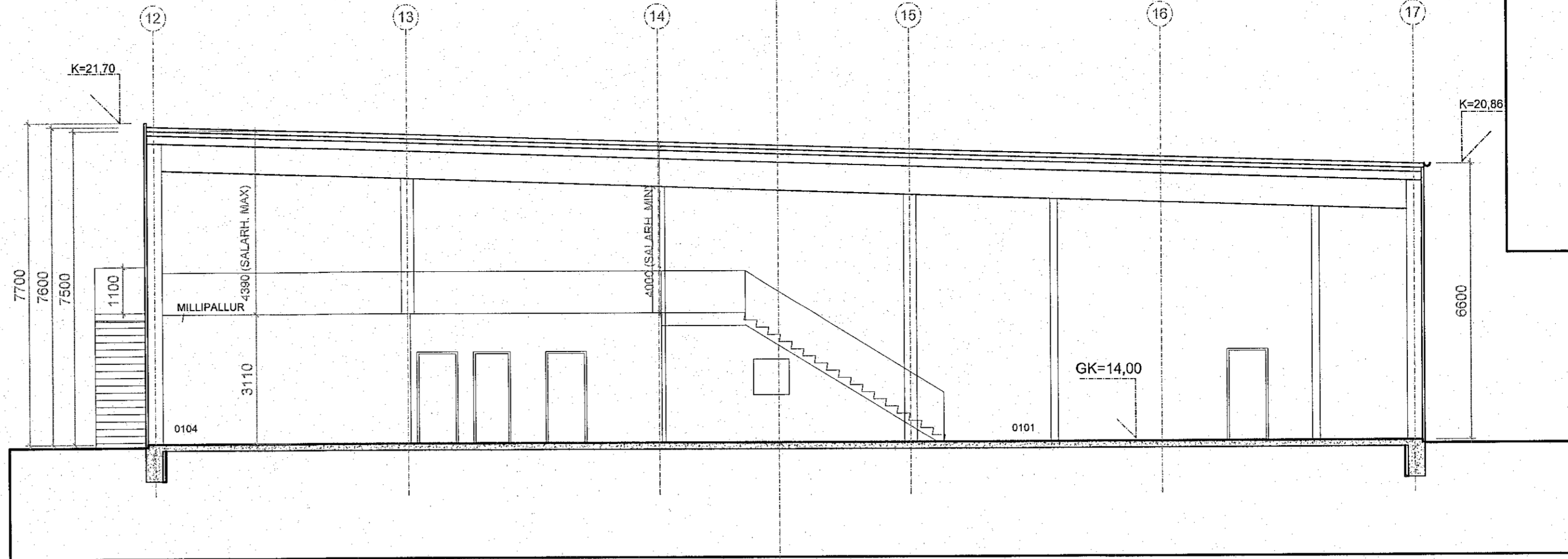
SNEIÐING D-D, NÝ VIÐBYGGING M1:100
