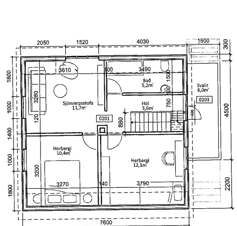
Grunnmynd rishæð Mkv. 1:100
