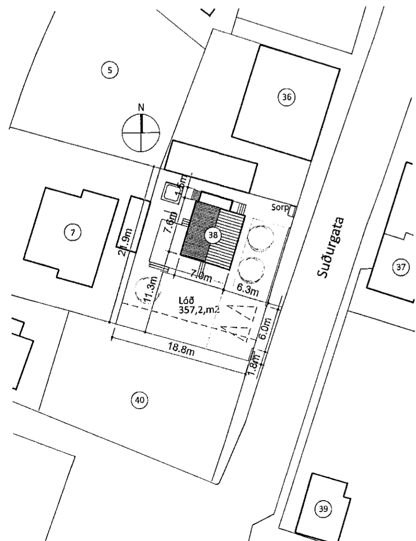
Afstöðumynd Mkv. 1:500
