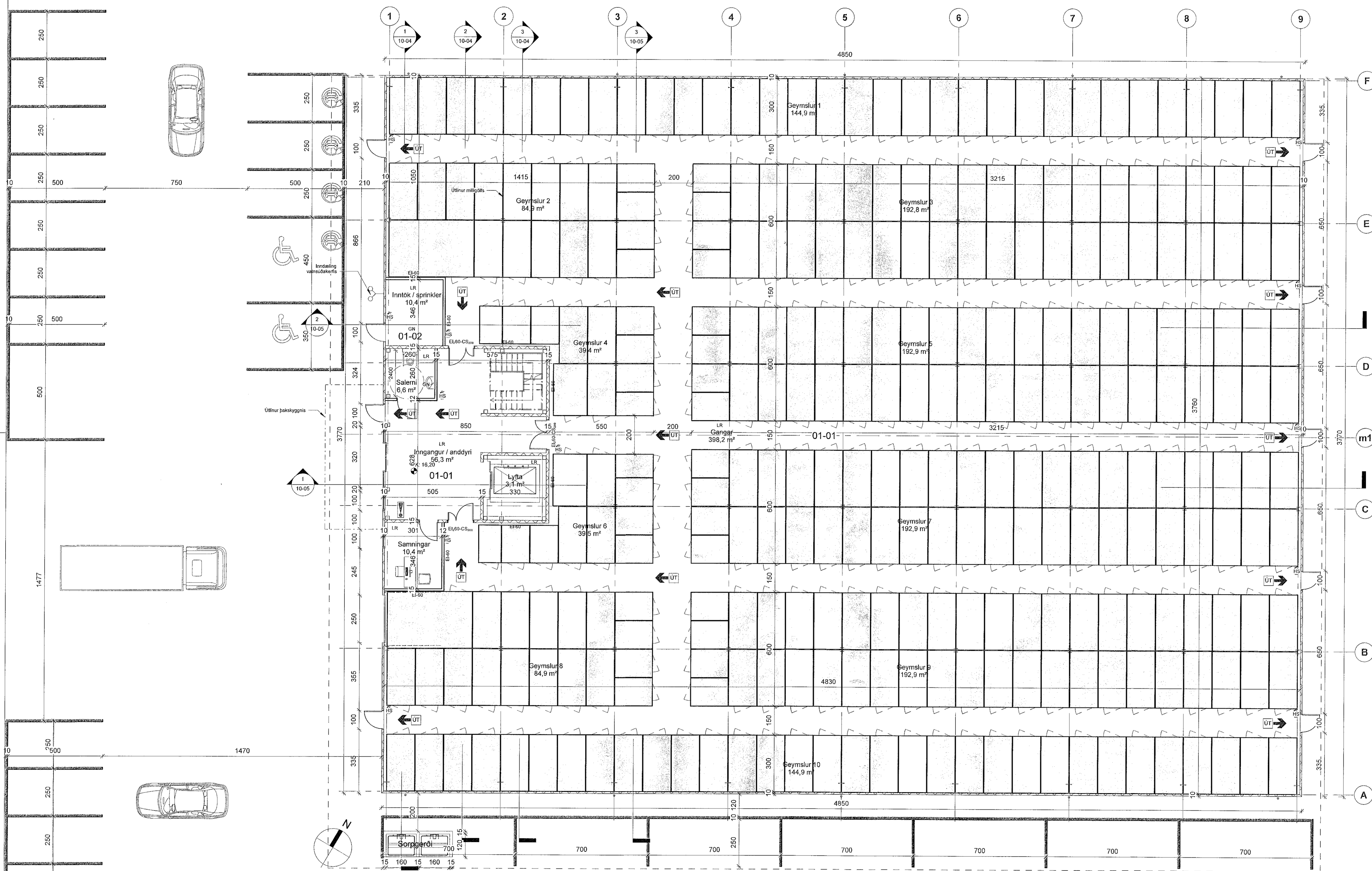
1 1. hæð 100 1:100
