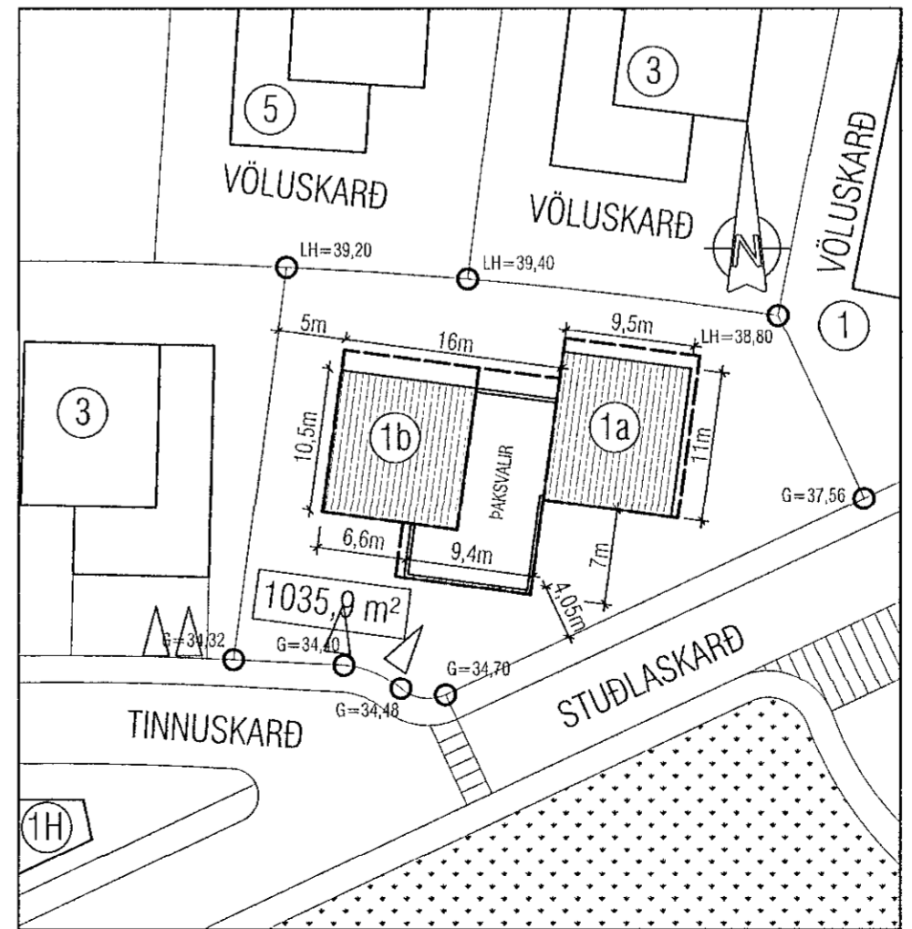
AFSTÖÐUMYND - 1:500
