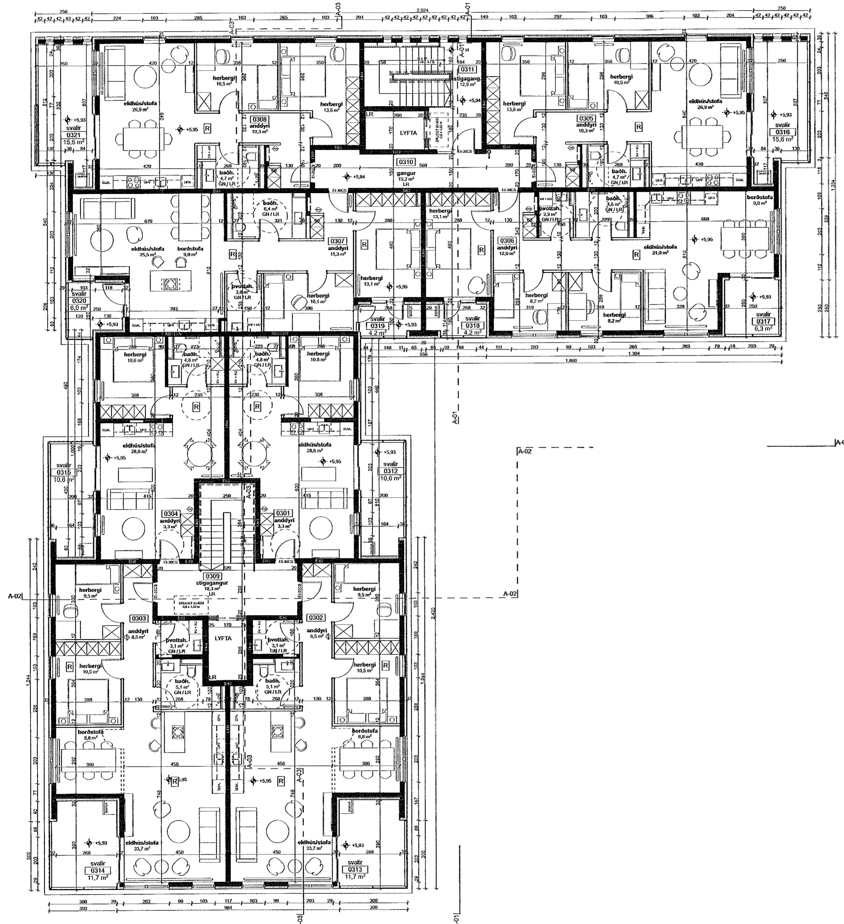
3.HÆÐ // 1:100
