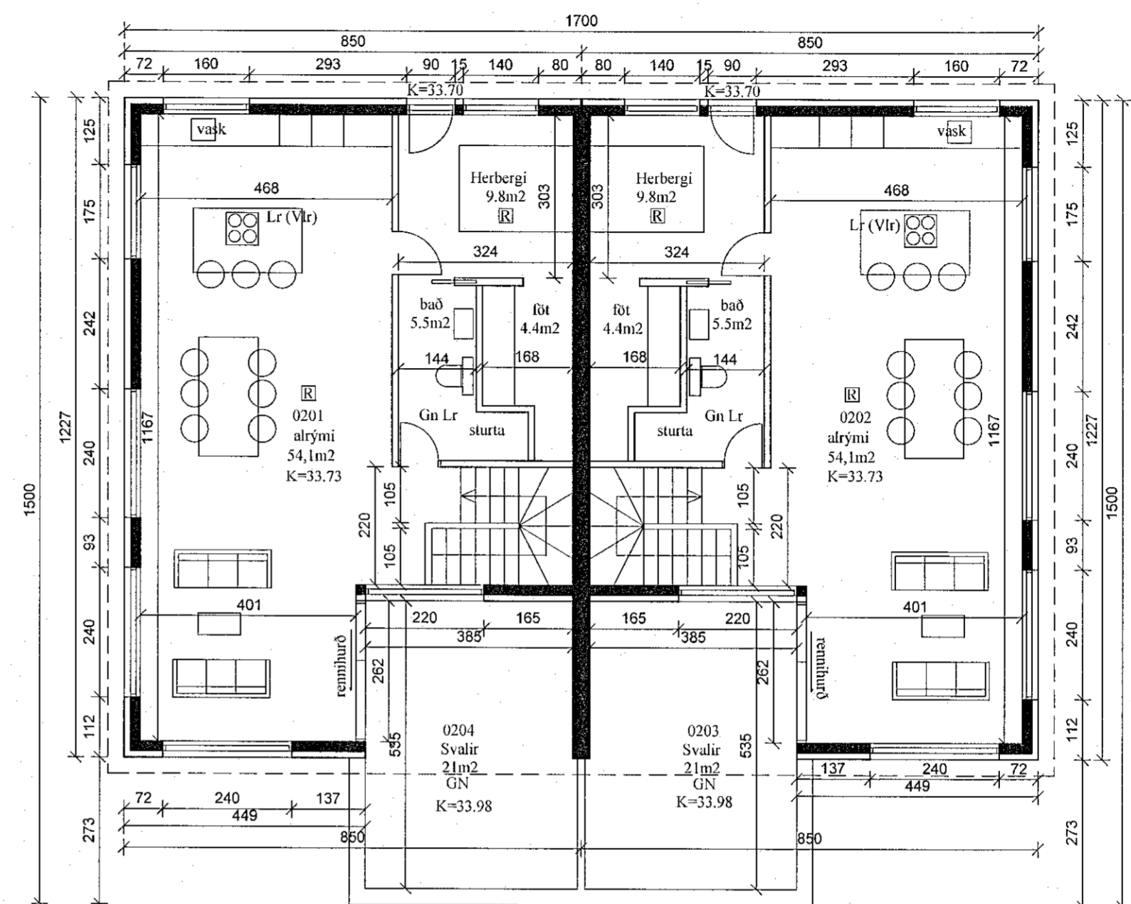
grunnmynd efri hæð
