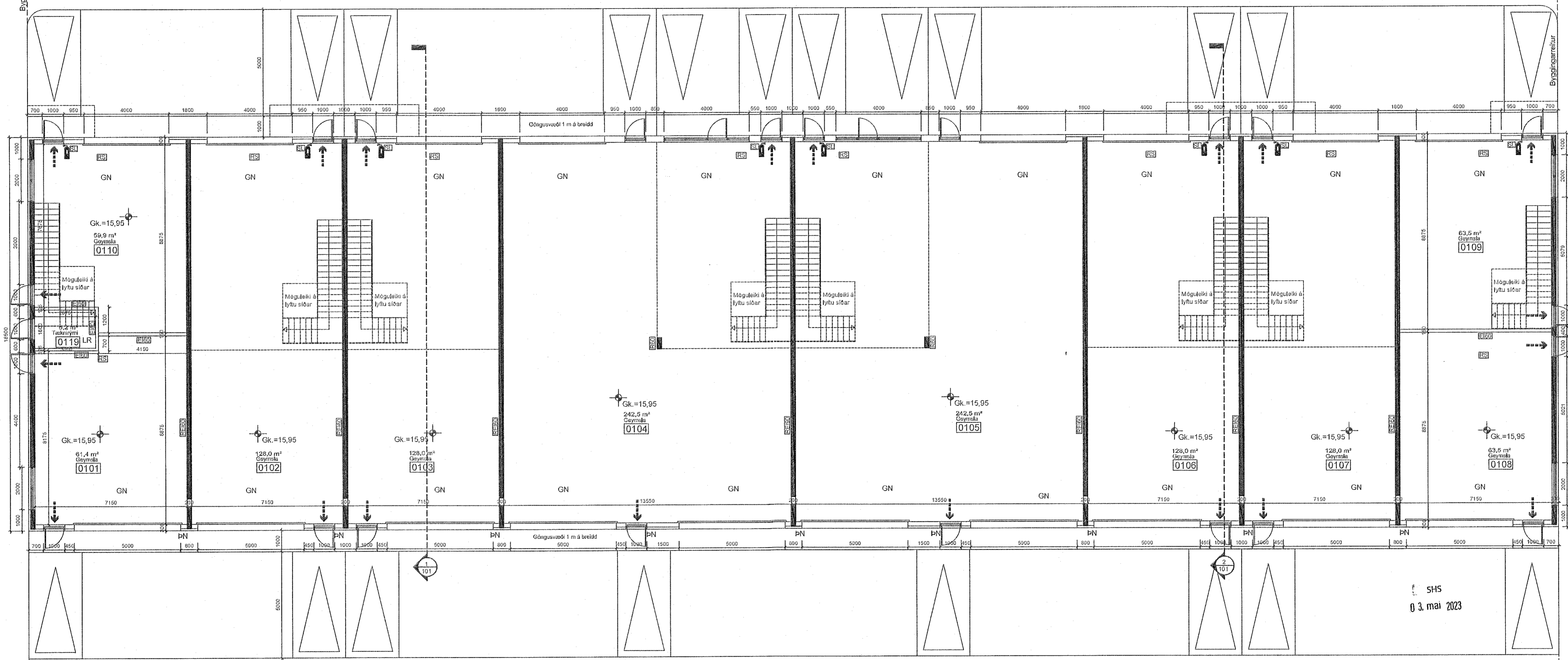
GRUNNMYND NEDRI HÆÐ mhl 02 1:100
