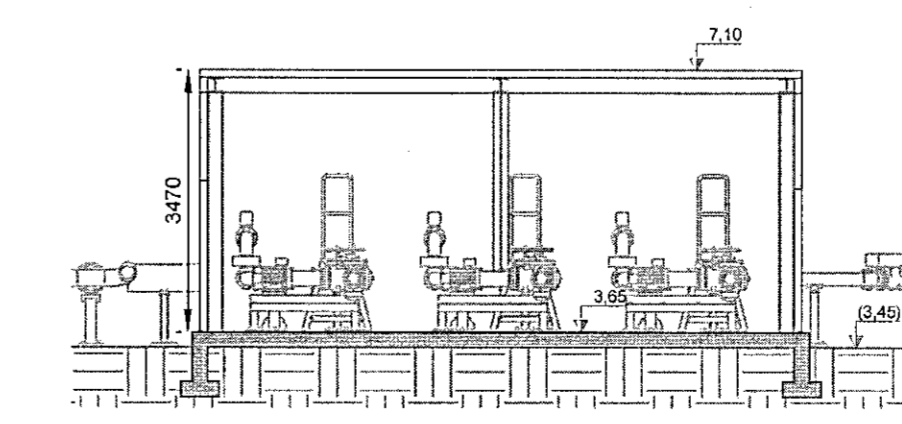
SNÍÐ B 1:100
