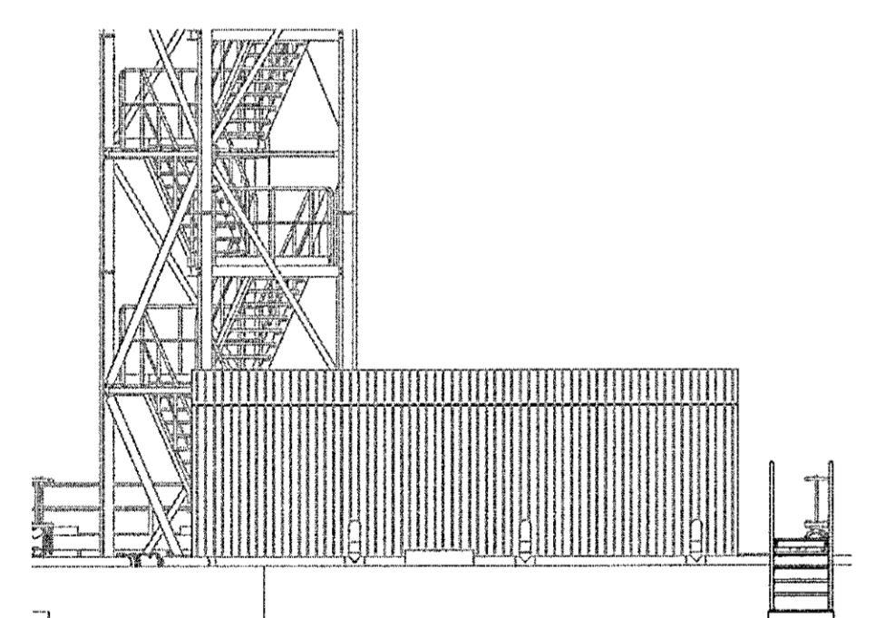
ÁSÝND - VESTURHLÍÐ 1:100
