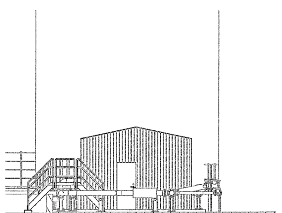
ÁSÝND - SÚÐURHLÍÐ 1:100
