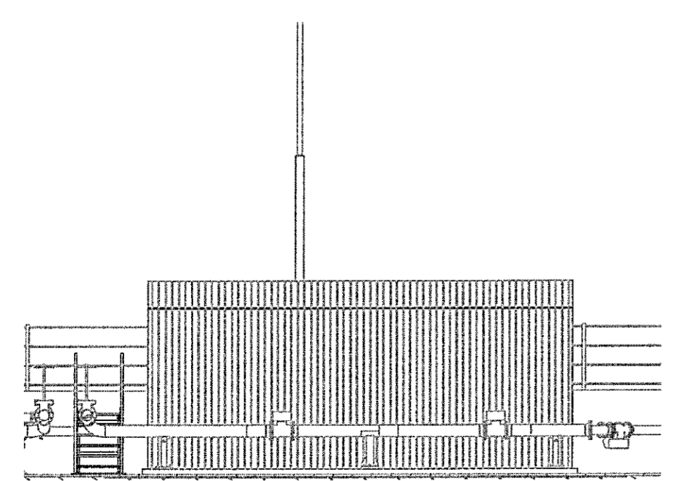
ÁSÝND - AUSTURHLÍÐ 1:100
