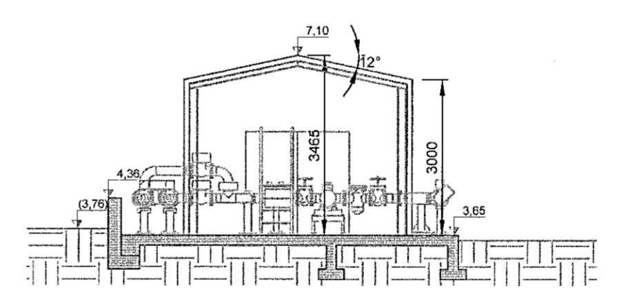
SNÍÐ A 1:100
