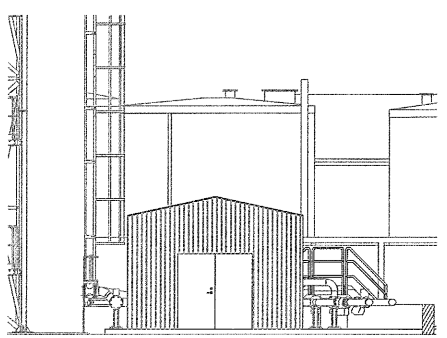
ÁSÝND - NORÐURHLÍÐ 1:100
