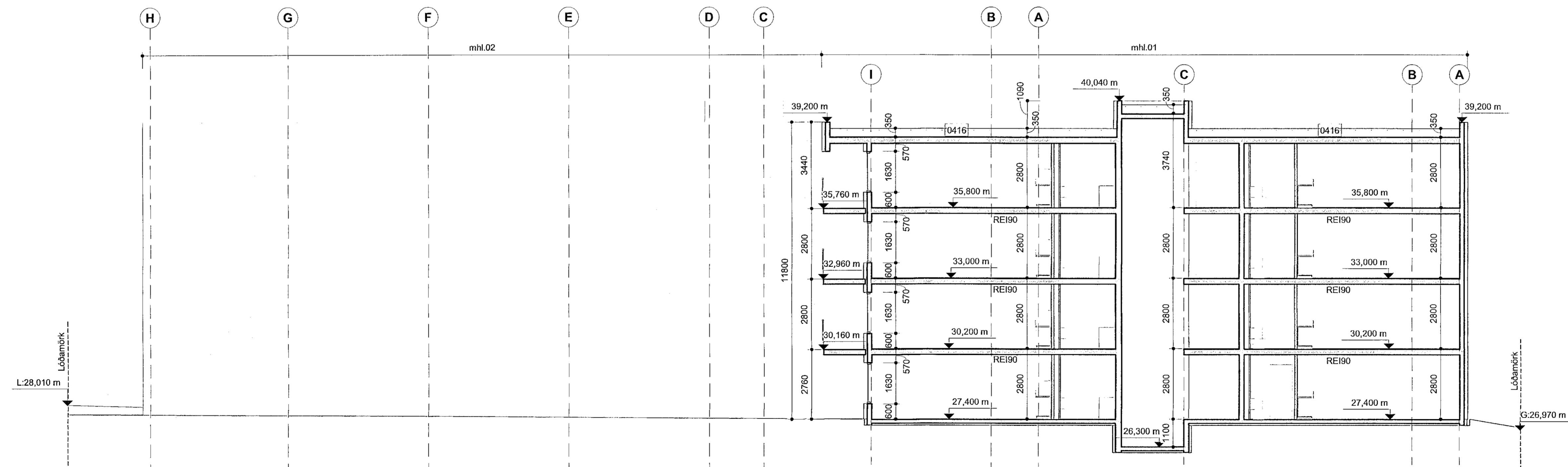
Snið D-D
