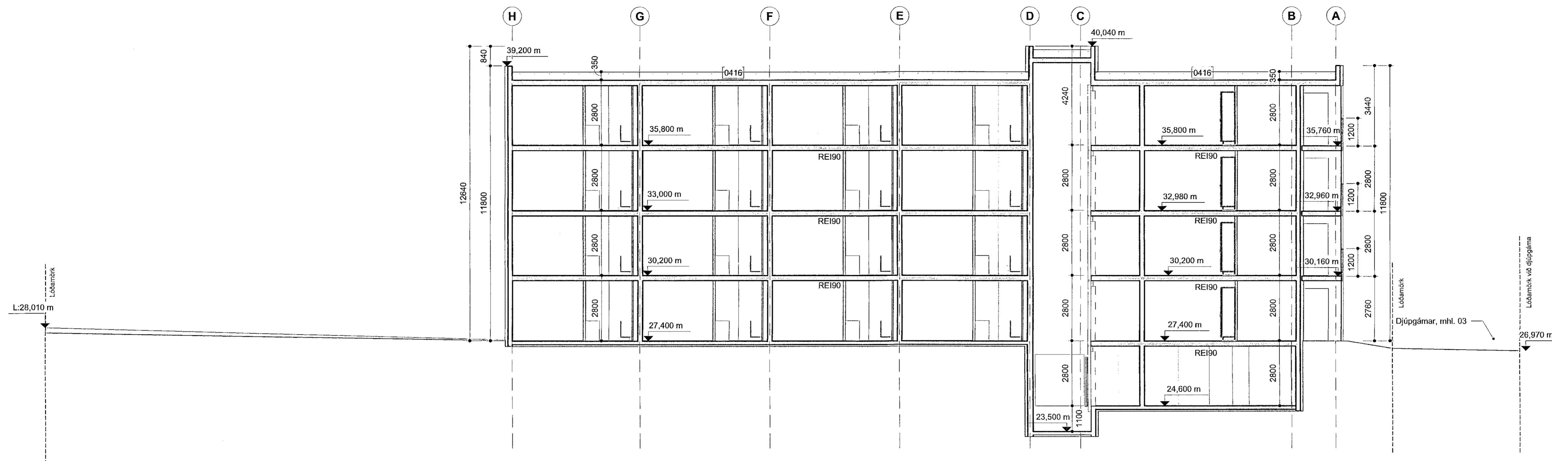
Snið C-C
