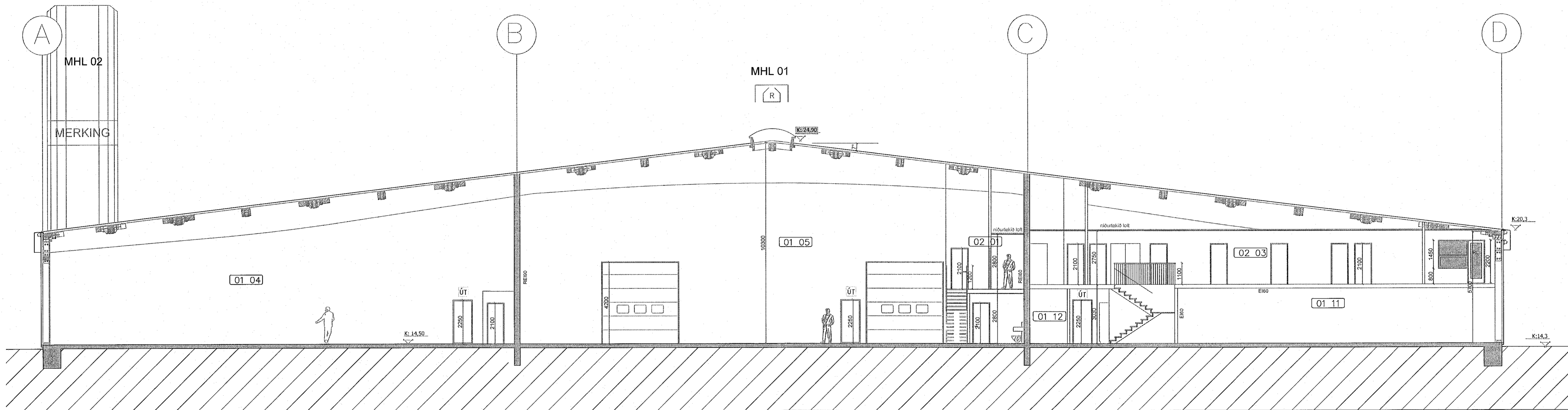
SNEIDING C-C 1:100
