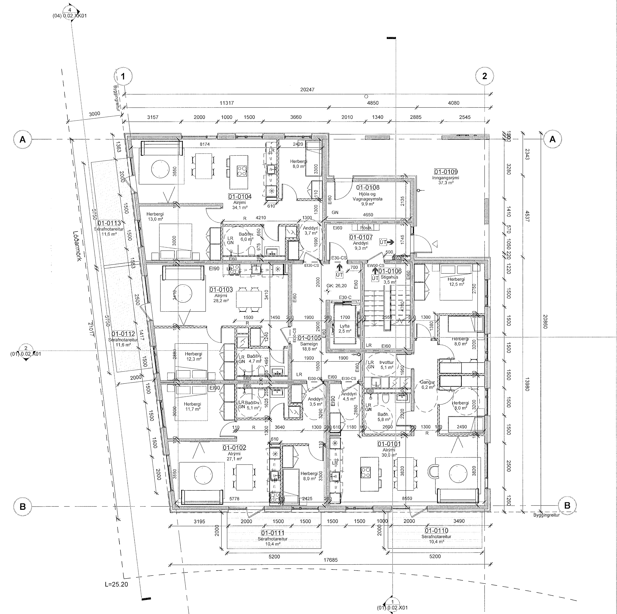
01-Hæð 1 - mhl 1 1: 100
